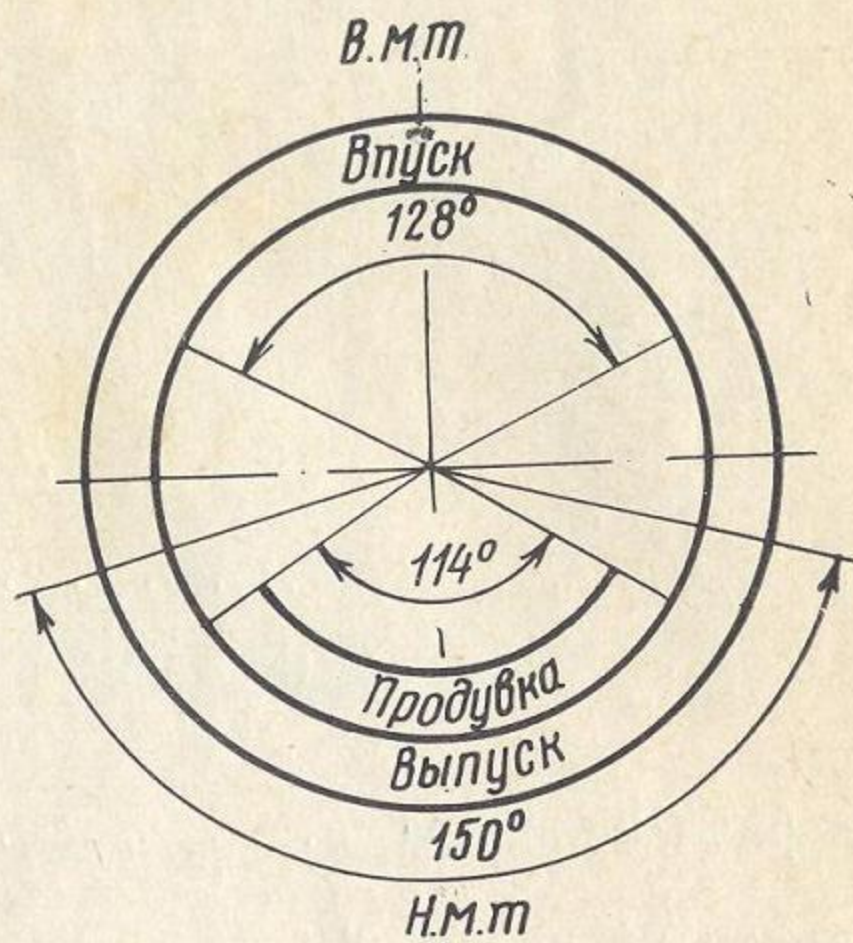
Фазы газораспределения двигателя «Восход»
