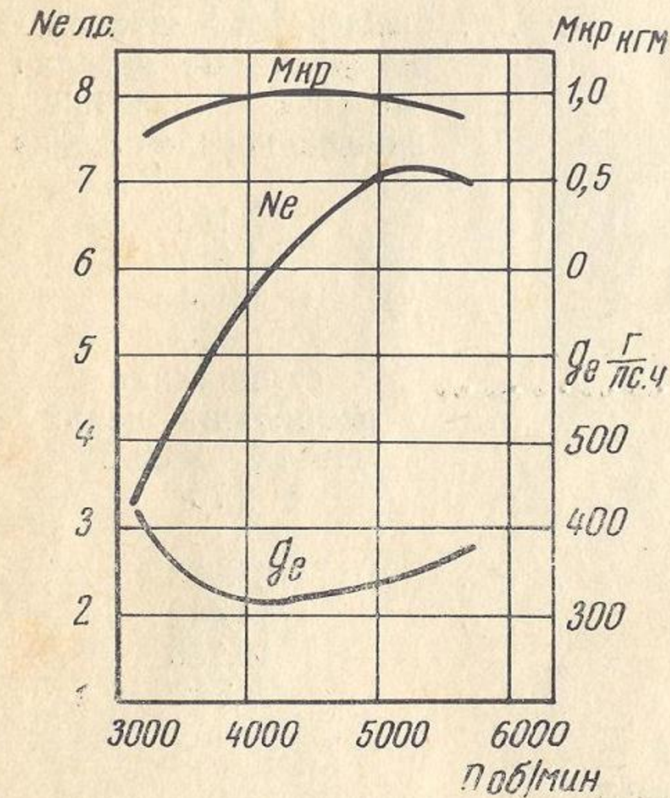
Скоростная характеристика двигателя М-105
