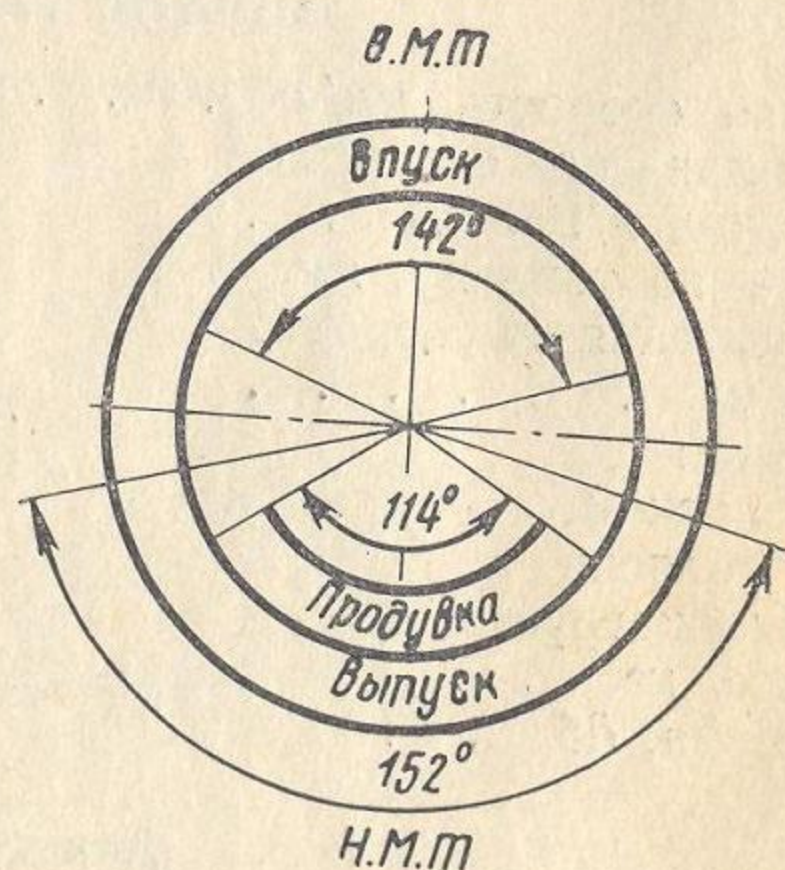
Фазы газораспределения двигателя ИЖ-Юпитер-2
