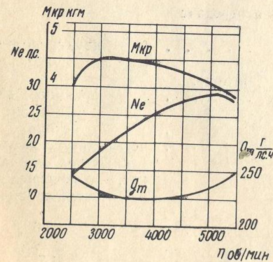
Скоростная характеристика двигателя М-63
