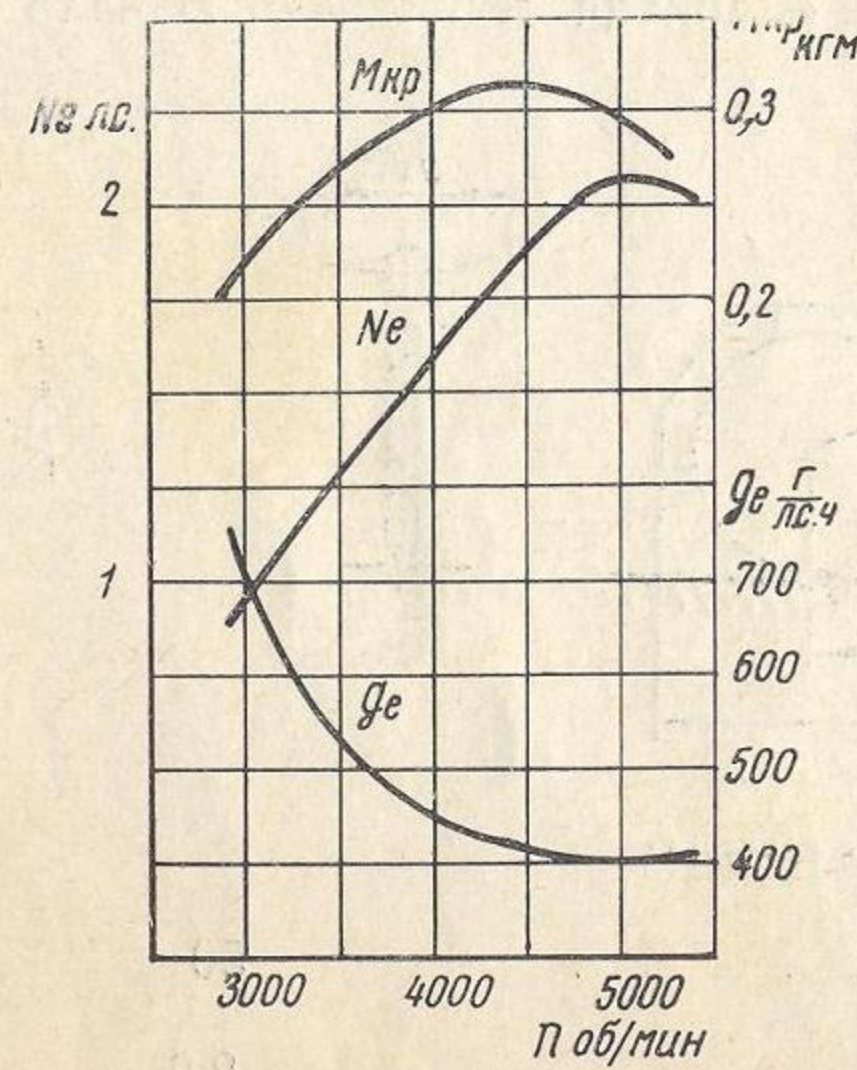
Скоростная характеристика двигателя Ш-51
