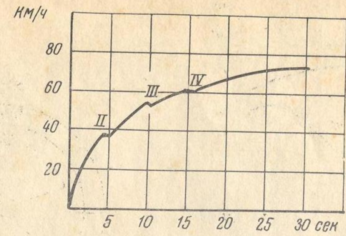
Время разгона мотороллера «Турист»
