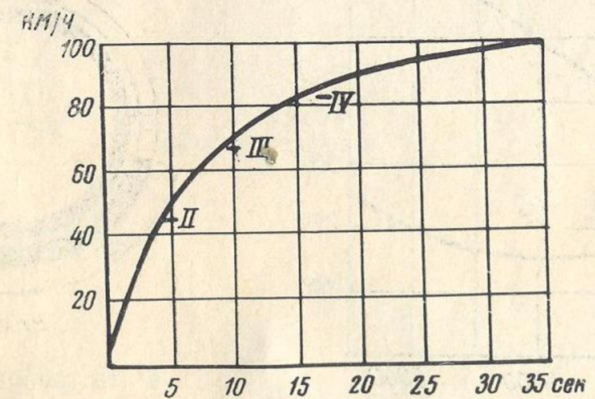
Время разгона мотоцикла К-650
