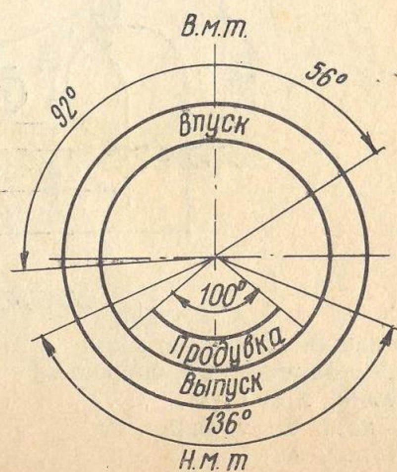
Фазы газораспределения двигателя Д-5
