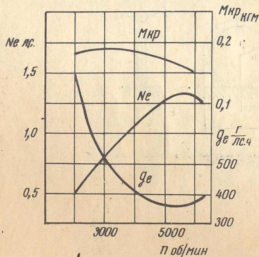
Скоростная характеристика двигателя Д-5
