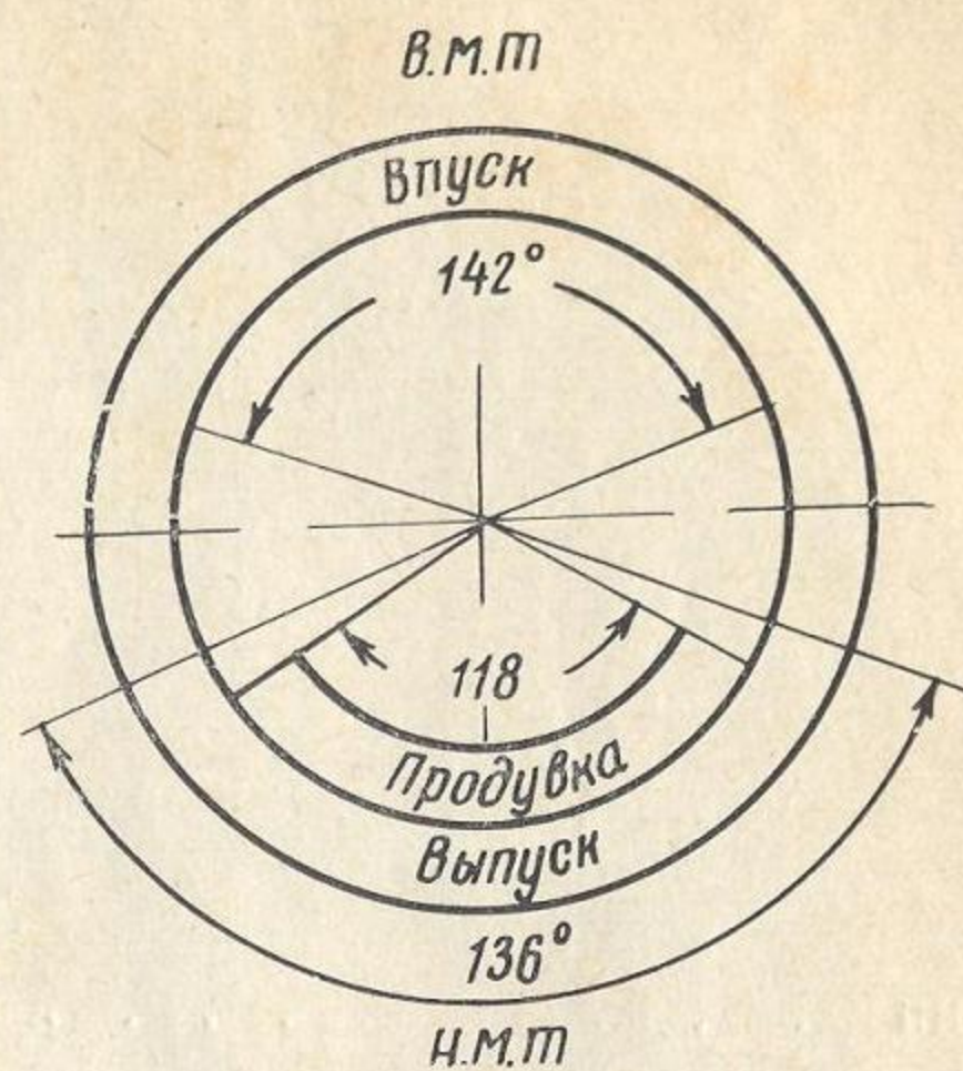
Фазы газораспределения двигателя В-150М
