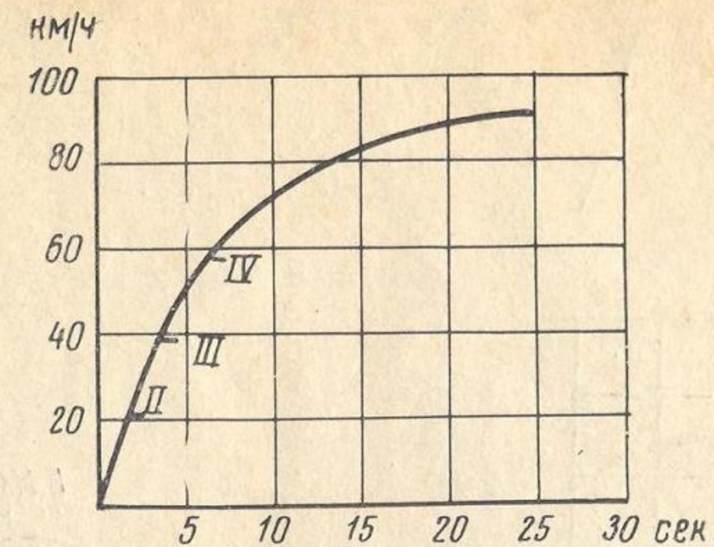
Время разгона мотоцикла «Восход»
