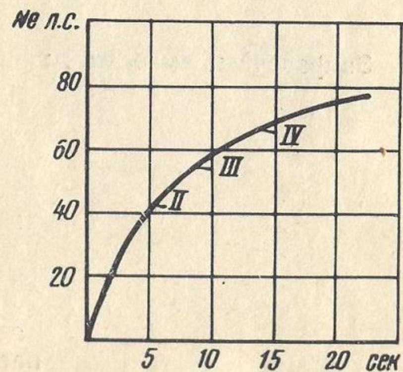
Время разгона мотоцикла К-750М
