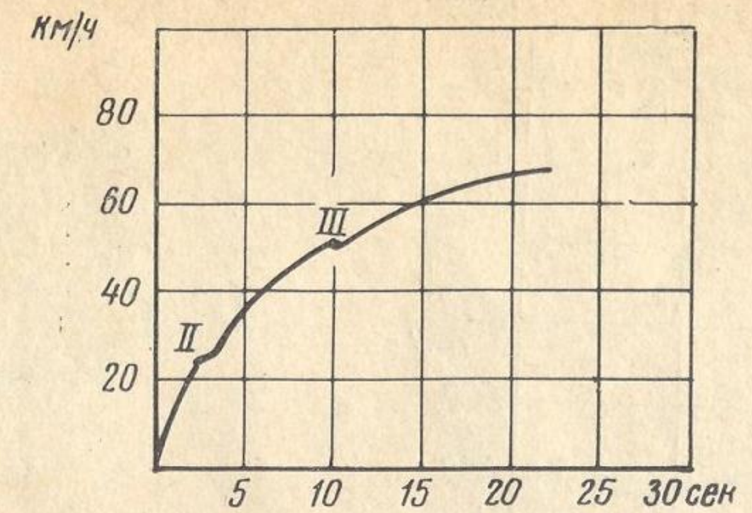
Время разгона мотороллера В150М
