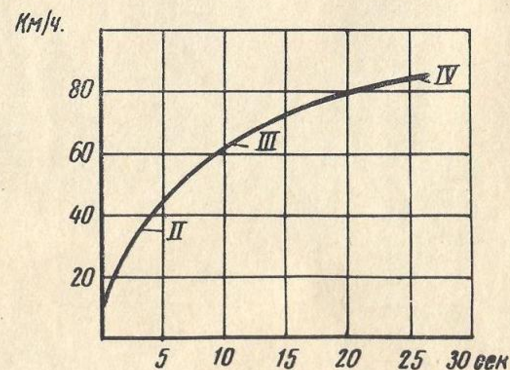
Время разгона мотоцикла М-63
