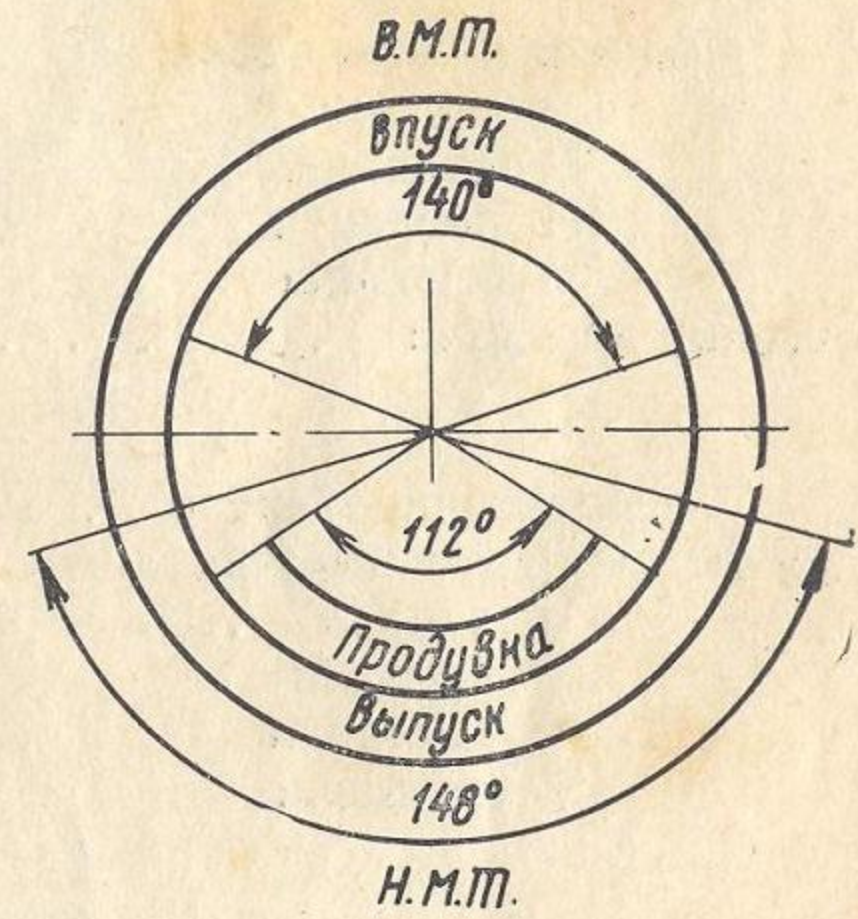
Фазы газораспределения двигателя М-105
