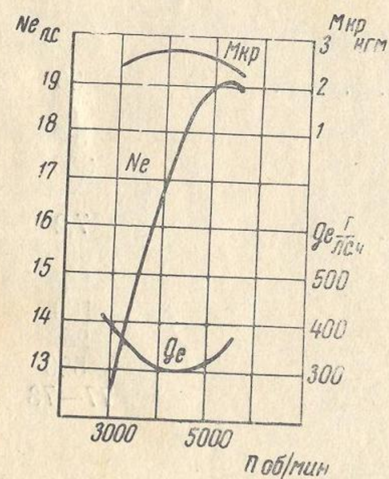
Скоростная характеристика двигателя ИЖ-Юпитер-2
