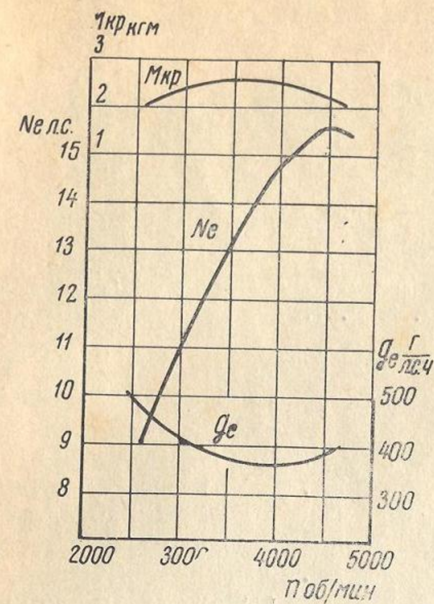
Скоростная характеристика двигателя ИЖ-Планета-2
