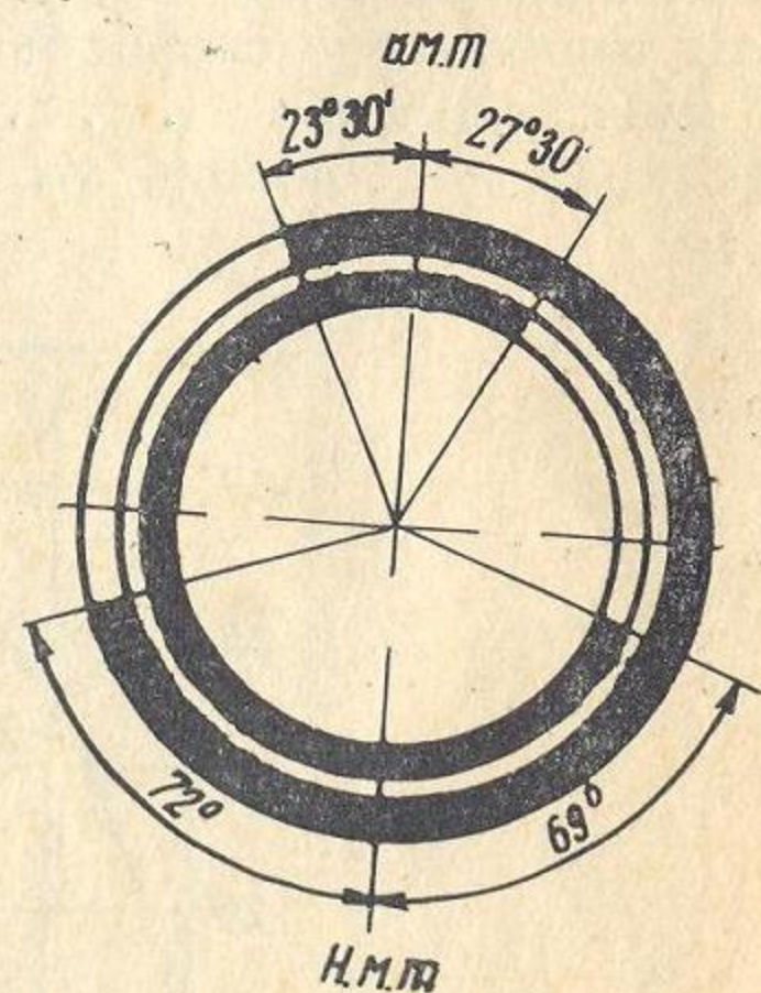
Фазы газораспределения двигателя К-650
