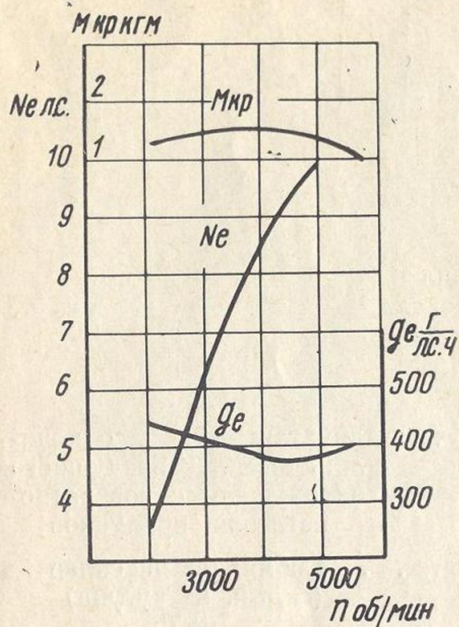
Скоростная характеристика двигателя «Восход»
