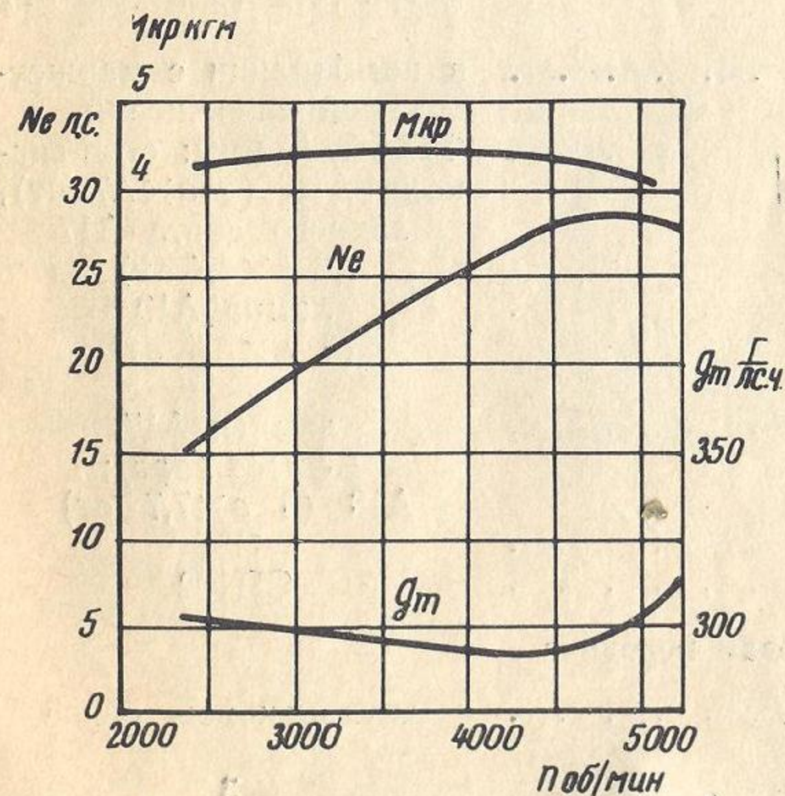
Скоростная характеристика двигателя К-750М
