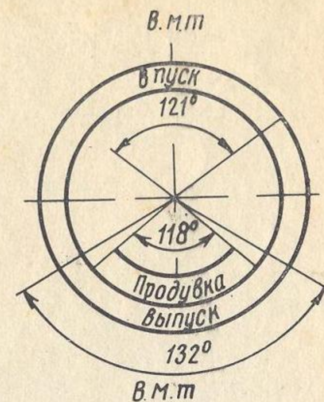
Фазы газораспределения двигателя ИЖ-Планета-2
