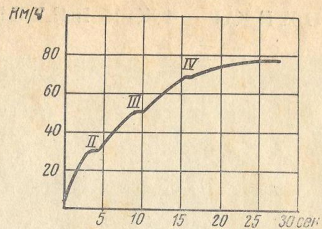
Время разгона мотоцикла ИЖ-Юпитер-2
