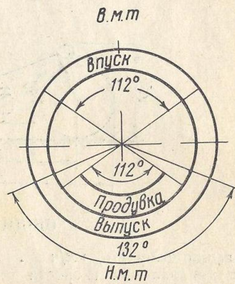
Фазы газораспределения двигателя Ш-51
