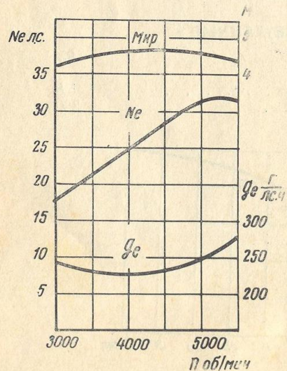
Скоростная характеристика двигателя К-650
