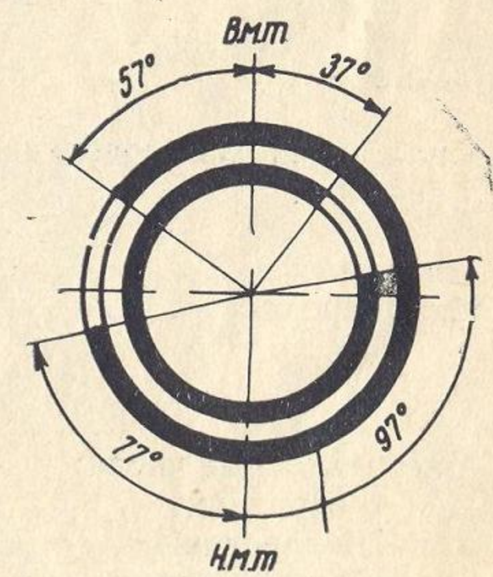
Фазы газораспределения двигателя М-63
