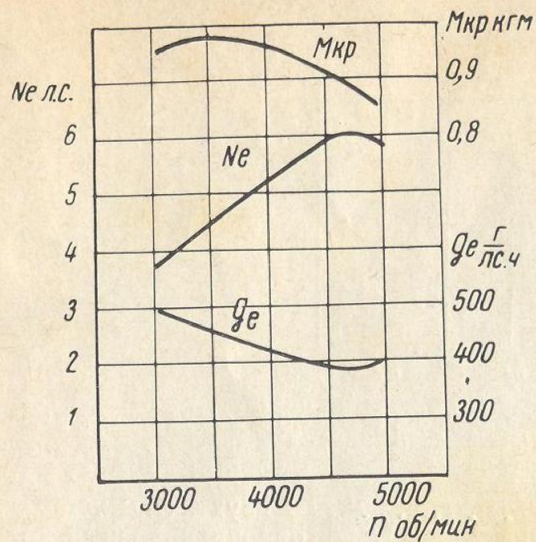
Скоростная характеристика двигателя В-150М
