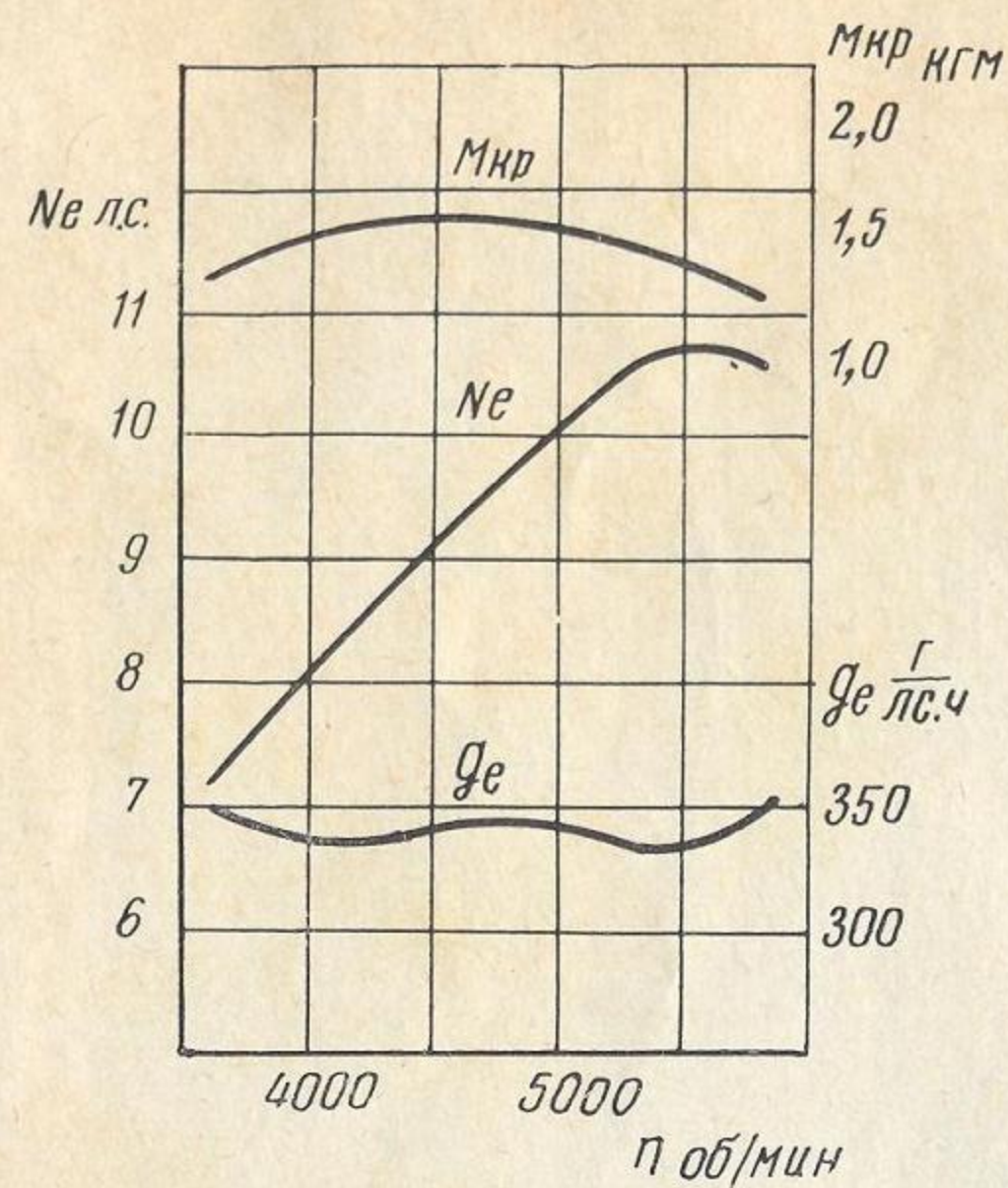
Скоростная характеристика двигателя «Турист»
