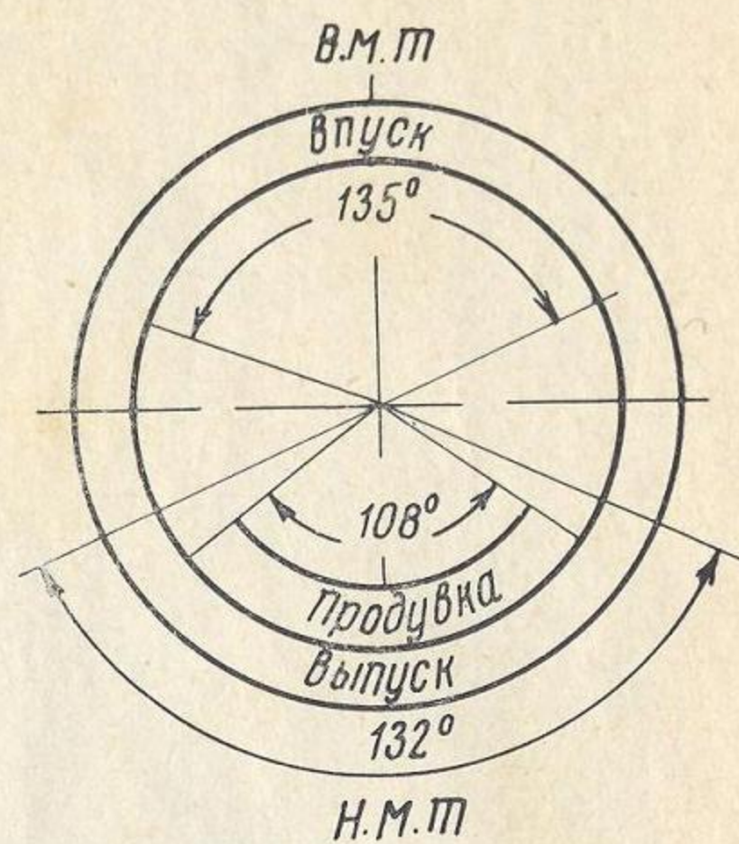
Фазы газораспределения двигателя «Турист»
