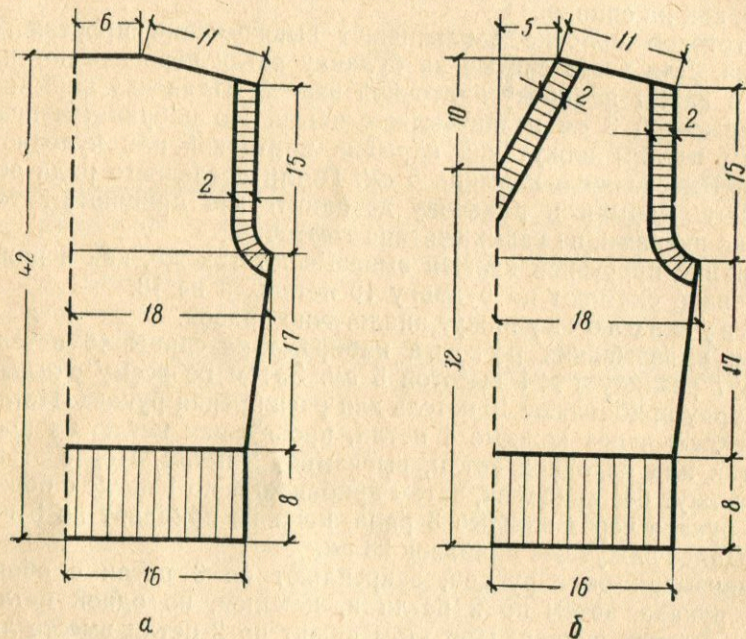
Рис. 75. Чертеж выкройки безрукавки для мальчика: а — спинка; б — перед
