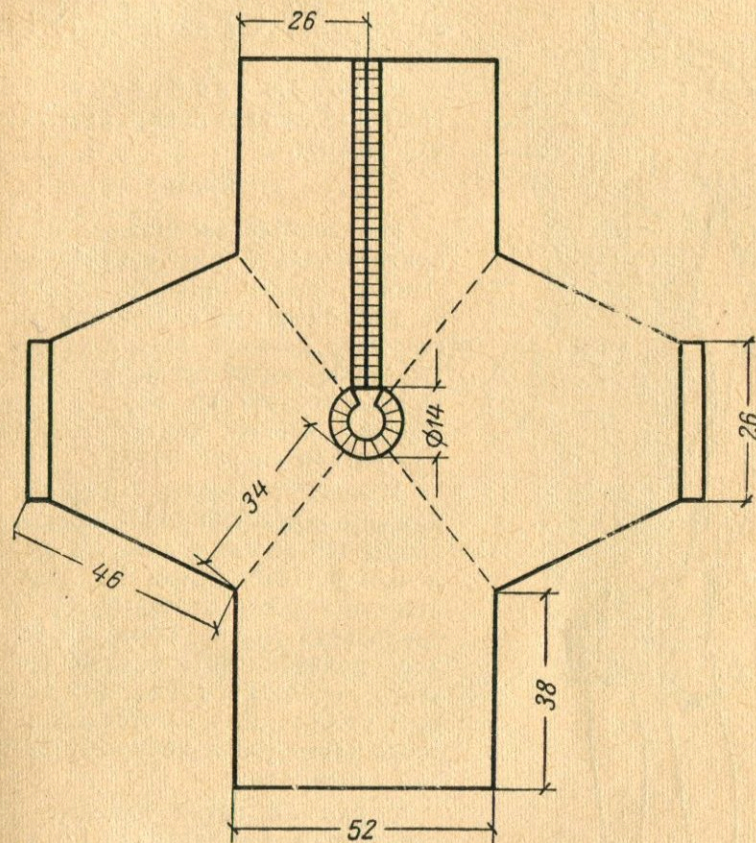
Рис. 115. Чертеж выкройки жакета, связанного на круговых спицах
