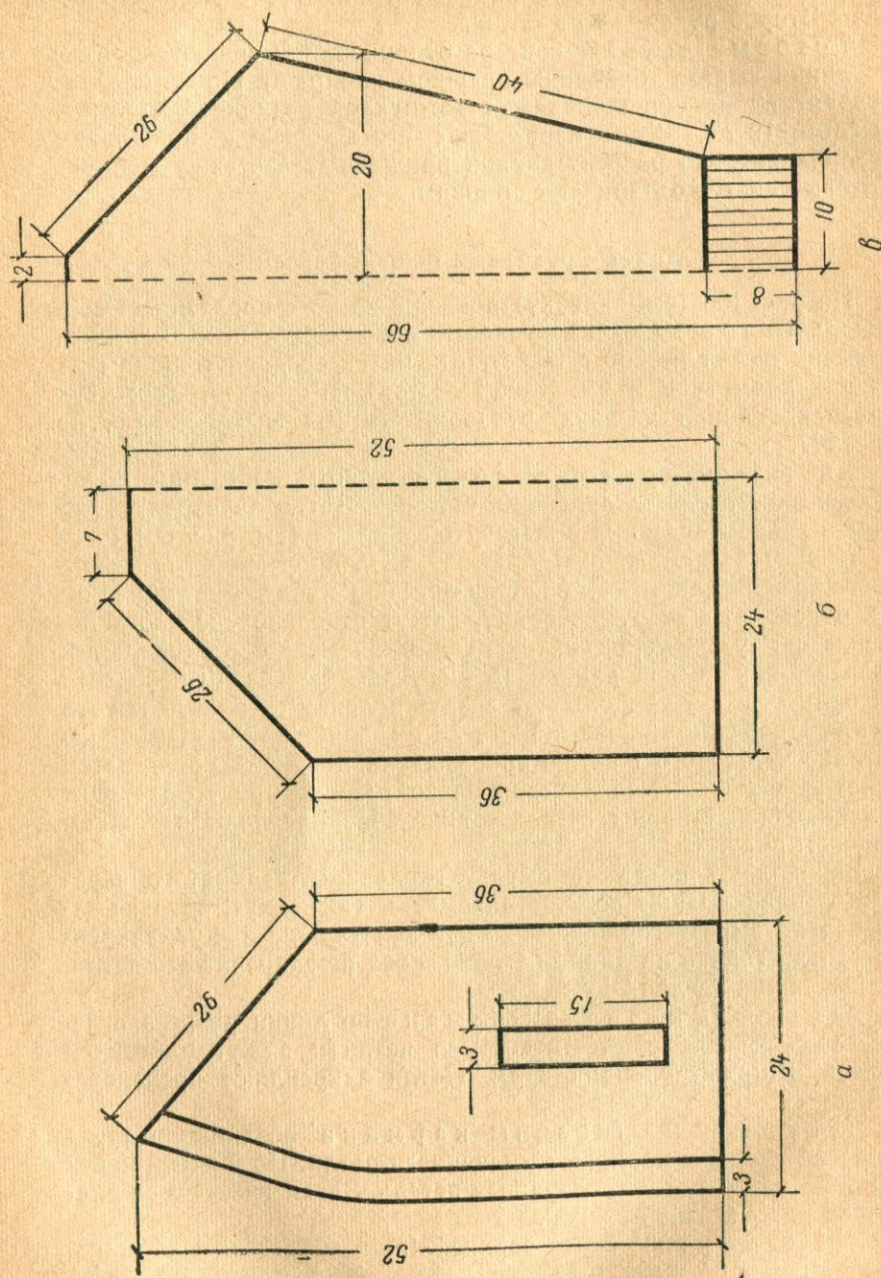
Рис. 107. Чертеж выкройки жакета с рукавами покрытием реглана: а — полочка; б — спинка; в — рукав
