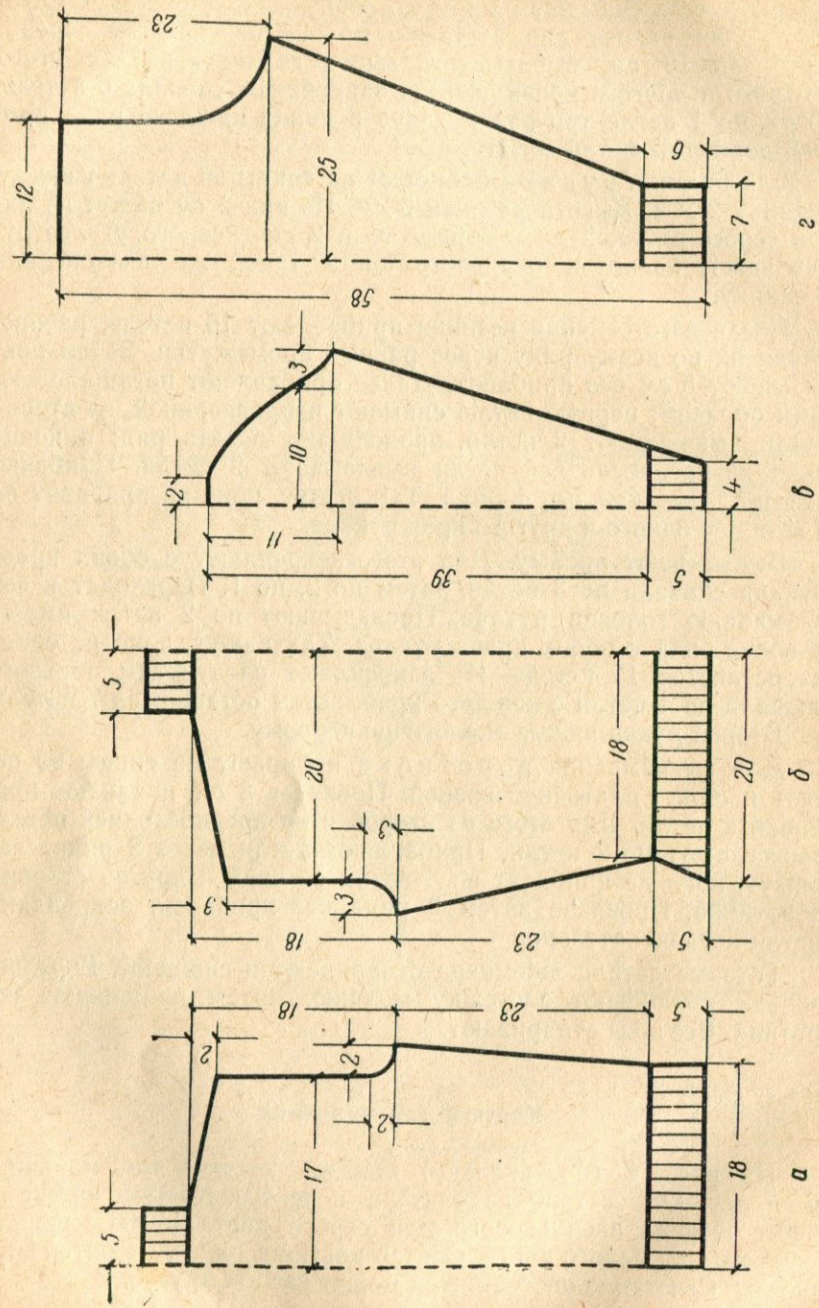
Рис. 79. Чертеж выкройки костюма для мальчишка: а — спинка; б — перед; в — рукав; г — рейтузы
