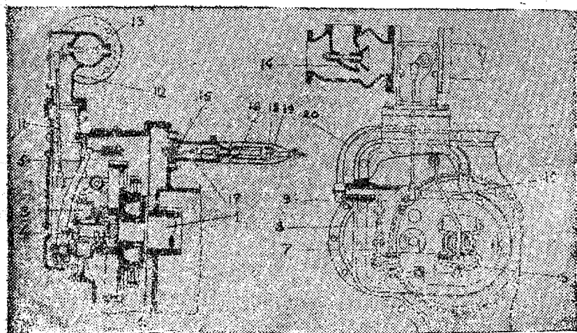
Рис. 24. Регулятор (продольный разрез и вид спереди): 1—распределительный вал; 2—шестерня распределительного вала; 3—грузик регулятора; 4—муфта регулятора; 5—рычаг регулятора длинный; 6—валик рычагов; 7—рычаг регулятора короткий; 8—тяги вилчатая; 9—рычаг дуплечи; 10—валик ограничителя; 11—тяги к дроссельной заслонке; 12—корпус дроссельной заслонки; 13—дроссельная заслонка; 14—смеситель; 15—пружина регулятора; 16—тяги пружины; 17—кронштейн-кожух; 18—регулировочная гайка; 19—контргайка; 20—наружный рычаг ограничителя.
