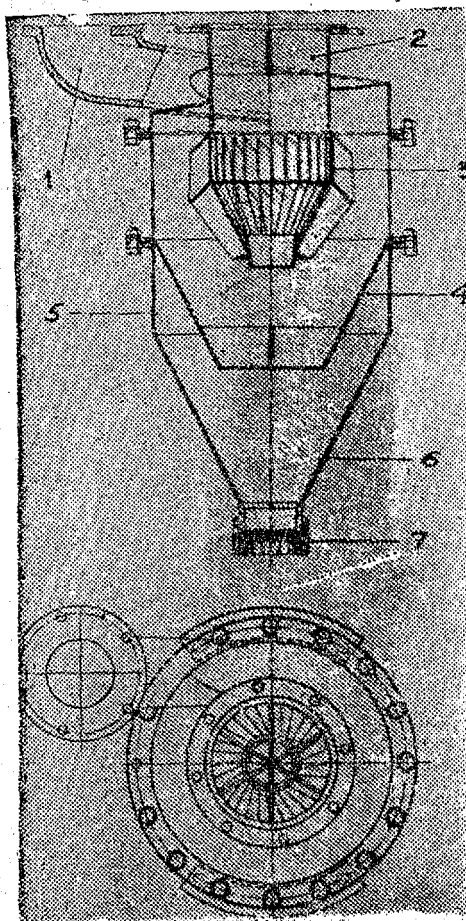
Рис. 16. Циклонный очиститель в сборе: 1—патрубок подвода газа; 2—патрубок вывода газа; 3—лопатки; 4—конус верхнего корпуса; 5—цилиндр нижнего корпуса; 6—конус нижнего корпуса; 7—пробка.
