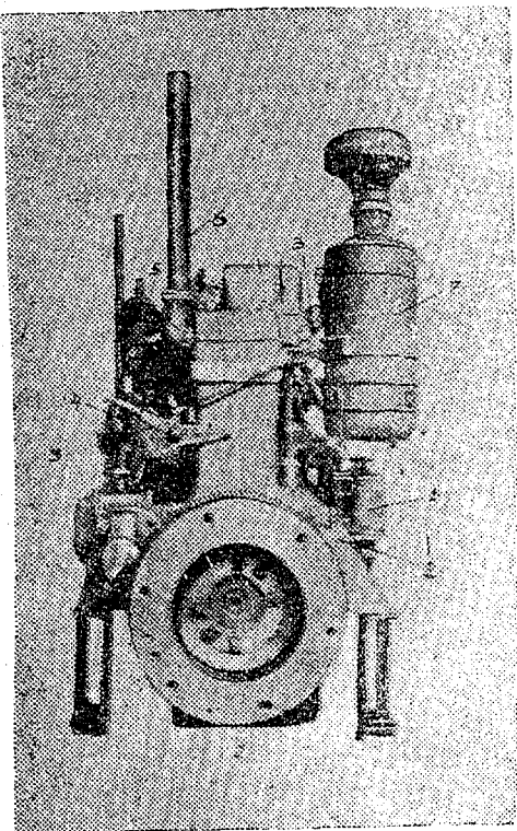
Рис. 23. Общий вид газового двигателя МГ—17 сзади: 1—маховик; 2—указатель; 3—механизм декомпрессора; 4—пусковой двигатель; 5—воздухоочиститель пускового двигателя; 6—выхлопная труба газового двигателя; 7—воздухоочиститель газового двигателя; 8—масляные фильтры.
