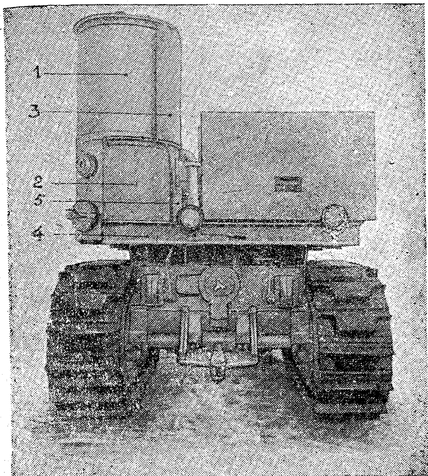
Рис. 8. Общий вид газогенераторной установки Г-25 на тракторе СГ-65 (вид сзади): 1—газогенератор; 2—опора газогенератора; 3—экран; 4—рама газогенератора; 5—факел газогенератора.
