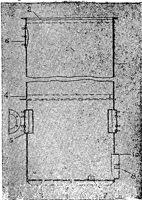
Рис. 10. Корпус газогенератора в сборе: 1—корпус; 2—фланец корпуса; 3—дно корпуса; 4—пояс крепления газогенератора; 5—коробка воздушного клапана; 6—фланец отбора газа; 7—упор для опоры колосниковой решетки; 8—ушко траверсы зольникового люка; 9—ребра жесткости днища; 10—горловина зольникового люка.
