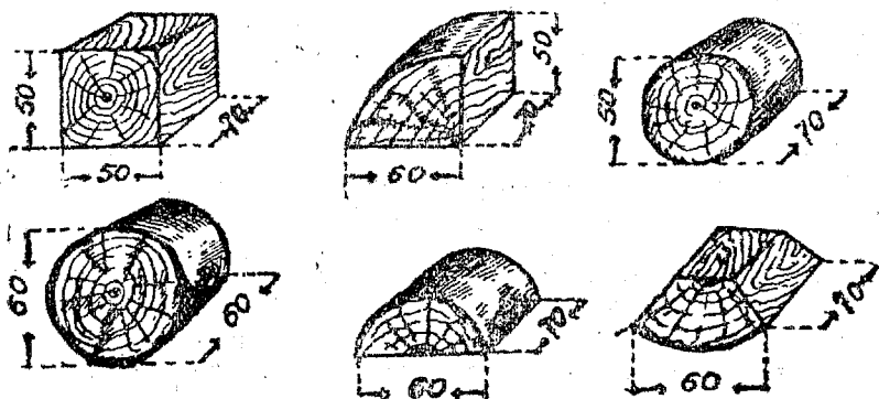
Рис. 4. Форма и размеры чурок (в мм) для трактора СГ—65.
