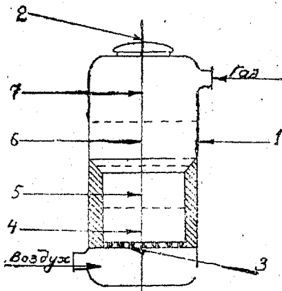
Рис. 1. Схема устройства газогенератора: 1 — корпус газогенератора; 2 — верхний (загрузочный) люк; 3 — колосниковая решетка; 4 — зона окисления или горения; 5 — зона восстановления; 6 — зона сухой перегонки; 7 — зона подсушки.
