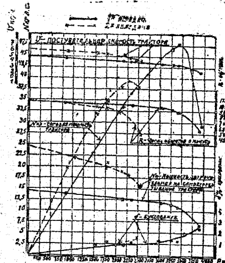
Рис. 45. Тяговые характеристики трактора СГ-65 (топливо — березовые чурки).
