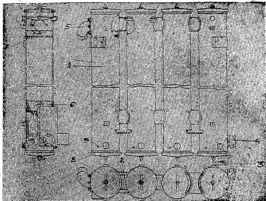
Рис. 18. Фильтр в сборе: 1—корпус цилиндра; 2—соединительные патрубки; 3—патрубок подвода газа; 4—пробка; 5—патрубок вывода газа; 6—коническая решетка опоры; 7—кольца Рашига; 8—крышки фильтра; 9—сливные трубки.
