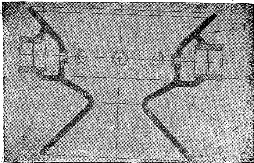
Рис. 13. Камера газификации газогенератора: 1—камера газификации; 2—формы камеры; 3—штуцер футорки.
