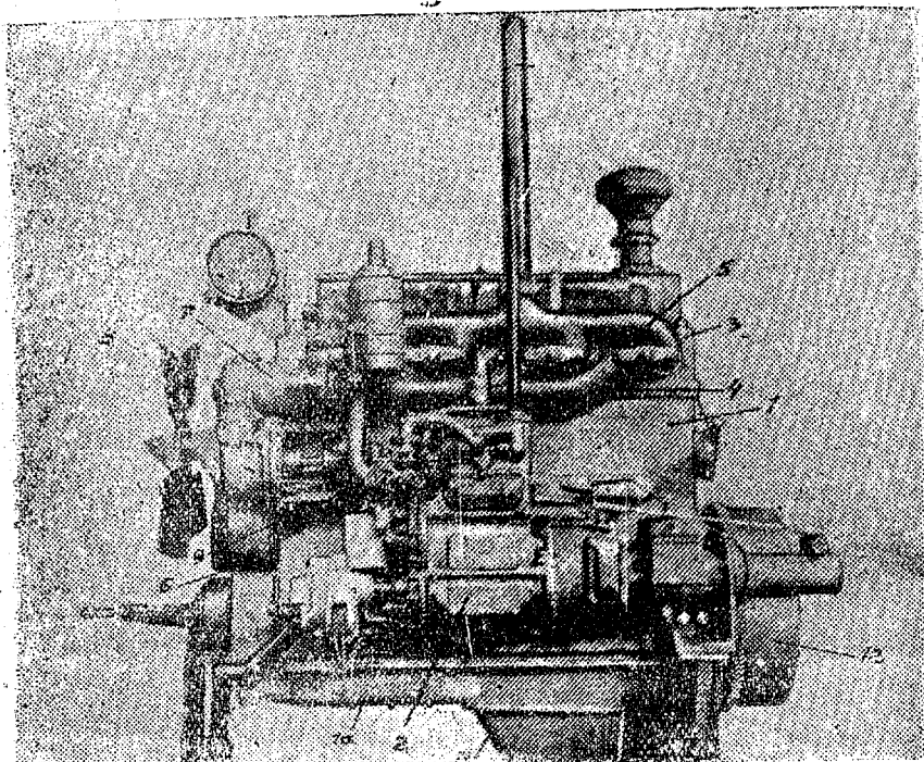
Рис. 21. Общий вид газового двигателя МГ-17 слева: 1—блок-картер; 2—пусковой двигатель; 3—головка блока; 4—всасывающая труба; 5—выхлопная труба; 6—кожух шестерен распределения; 7—динамо; 8—вентилятор; 9—водяной насос; 10—нижний картер; 11—поддон; 12—маховик.
