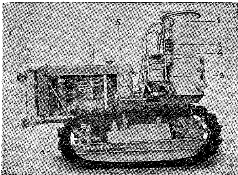
Рис. 6. Общий вид газогенераторной установки Г—25 на тракторе СТЗ—65 (вид слева): 1—газогенератор; 2—компенсатор; 3—циклонный очиститель; 4—загрузочная площадка; 5—пластинчатые очистители; 6—газопровод от пластинчатого очистителя к фильтру; 7—фильтр газа.
