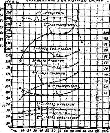
Рис. 44. Кривые мощности температур и разрежений при выжиге топлива в газогенераторе Г-25 (топливо — березовые чурки).
