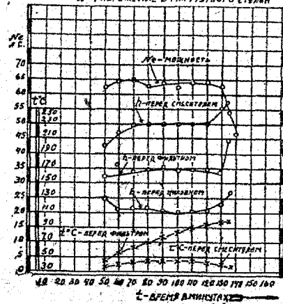
Рис. 44. Кривые мощности температур и разрежений при выжиге топлива в газогенераторе Г-25 (топливо — березовые чурки).
