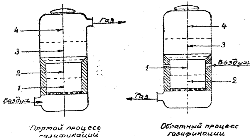
Рис. 2. Схема прямого и обратного процесса газификации: 1—зона окисления или горения; 2—зона восстановления; 3—зона сухой перегонки; 4—зона подсушки.
