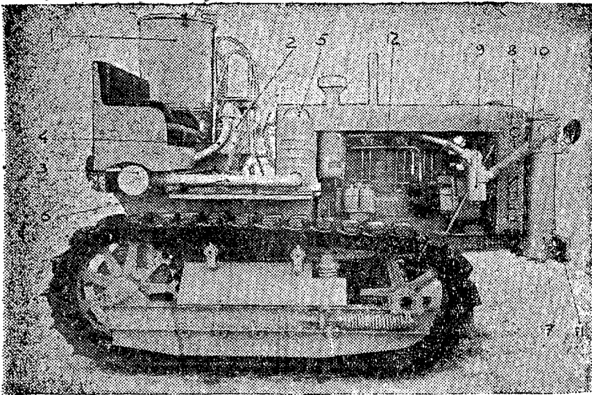
Рис. 5. Общий вид газогенераторной установки Г-25 на тракторе СГ-65 (вид справа): 1—газогенератор; 2—циклонный очиститель; 3—первый цилиндр пластинчатого очистителя; 4—газопровод от циклонов к первому цилиндру пластинчатого очистителя; 5—второй, третий и четвертый цилиндры пластинчатого очистителя; 6—газопровод от первого ко второму цилиндру пластинчатого очистителя; 7—фильтр; 8—радиатор двигателя; 9—отстойник; 10—соединительный шланг отстойника с фильтром; 11—бампер; 12—газовый двигатель.
