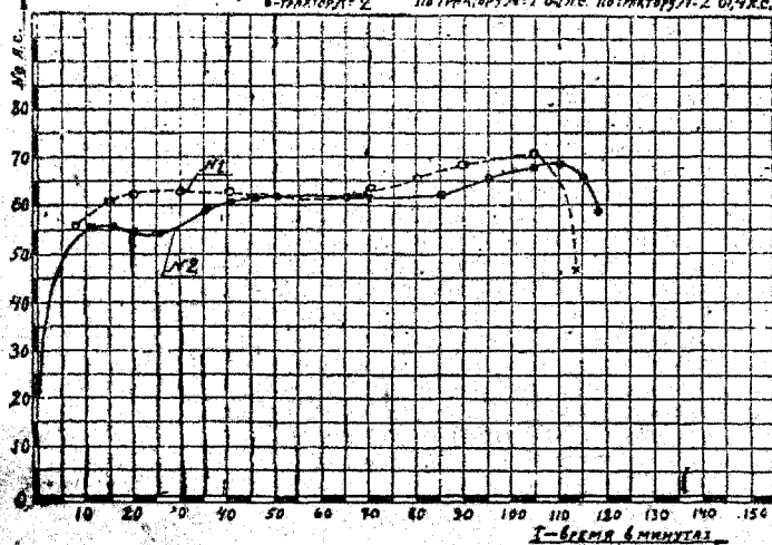
Рис. 43. Кривая мощности газового двигателя МГ-17 при выжиге топлива в газогенераторе Г-25 (топливо — березовые чурки).
