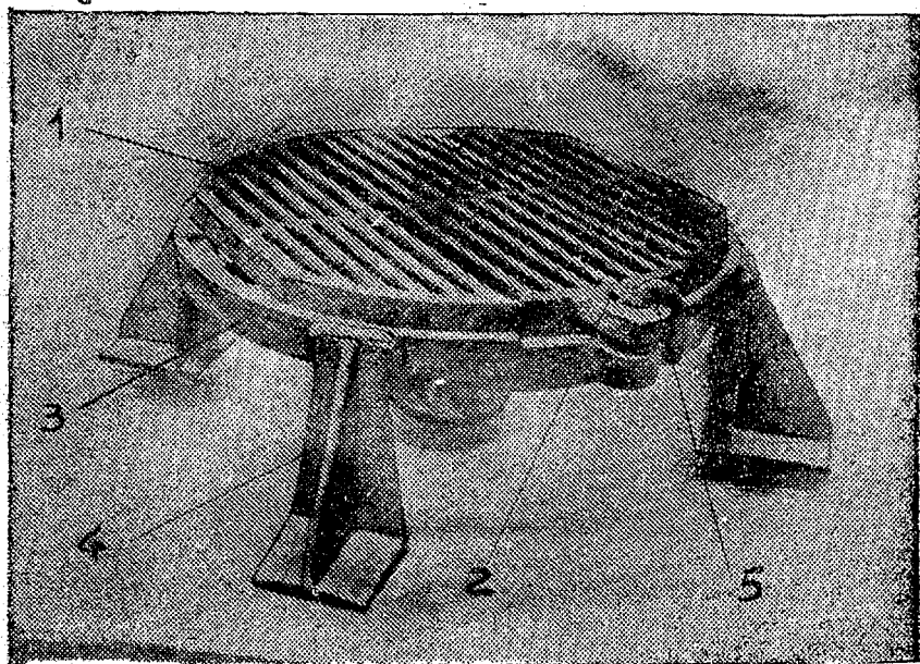
Рис. 14. Колосниковая решетка в сборе: 1—боковые секции колосниковой решетки; 2—средняя секция колосниковой решетки; 3—опорное кольцо; 4—стойки опорного кольца; 5—замок колосниковой решетки.
