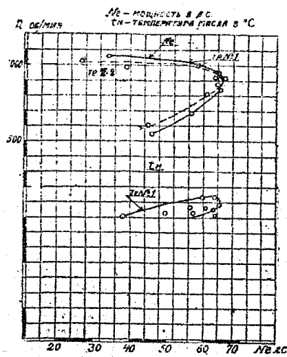
Рис. 41. Регуляторная характеристика газового двигателя МГ-17 (топливо — березовые чурки).
