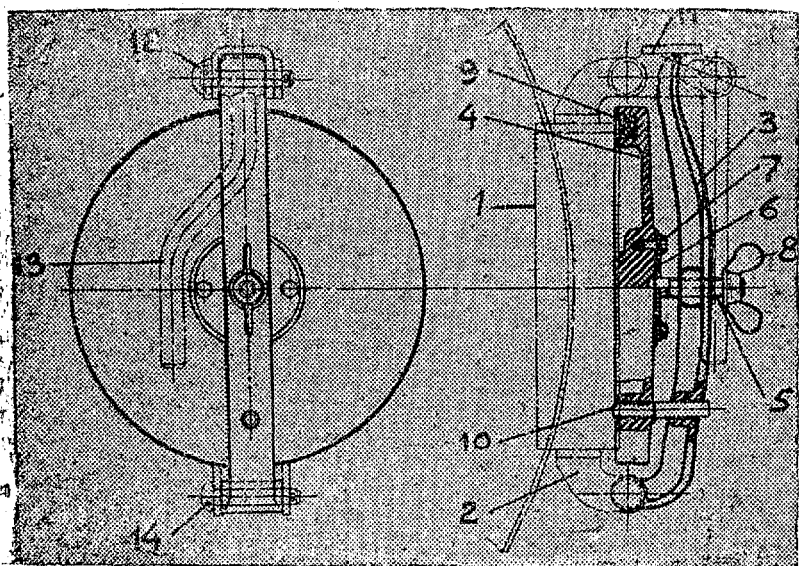
Рис. 11. Крышка зольникового люка газогенератора в сборе: 1—горловина; 2—ушко горловины; 3—траверса крышки; 4—крышка; 5—упорный винт крышки; 6—шайба упорного винта крышки; 7—болт шайбы упорного винта; 8—барашек упорного винта крышки; 9—прокладка крышки; 10—установочная шпилька траверсы; 11—серьга запорного рычага крышки; 12—палец серьги; 13—запорный рычаг крышки; 14—палец запорного рычага крышки.
