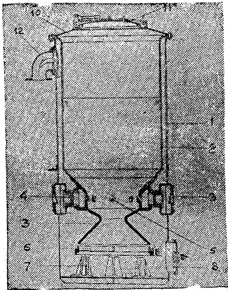
Рис. 9. Газогенератор в сборе: 1—корпус газогенератора; 2—бункер газогенератора; 3—камера газификации (горения) газогенератора; 4—фурторки газогенератора; 5—фурмы камеры горения; 6—колосниковая решетка; 7—опора колосниковой решетки, 8—зольниковый люк; 9—воздушные клапаны; 10—крышка газогенератора; 11—загрузочный люк газогенератора; 12—патрубок отбора газа.
