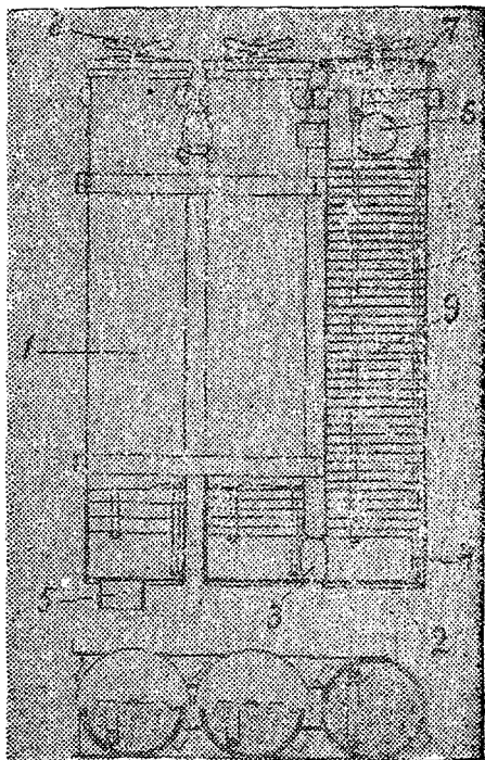
Рис. 17. Пластинчатый очиститель в сборе: 1—корпус цилиндра; 2—дно цилиндра; 3—соединительный патрубок; 4—соединительные шпильки; 5—патрубок ввода газа; 6—патрубок вывода газа; 7—крышка; 8—барашек; 9—секции пластинчатых очистителей.
