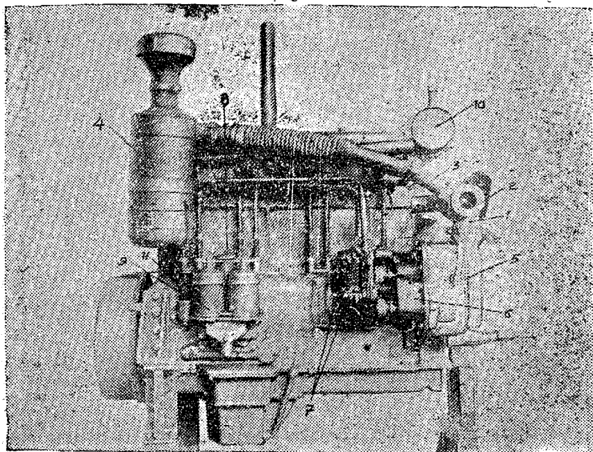
Рис. 20. Общий вид газового двигателя МГ—17 справа: 1—корпус дроссельной заслонки; 2—смеситель; 3—патрубок подвода воздуха к смесителю; 4—воздухоочиститель; 5—кожух шестерен распределения; 6—кронштейн магнето; 7—магнето; 8—маслоналивная горловина; 9—масляные фильтры; 10—бензиновый бачек пускового двигателя; 11—свечи.
