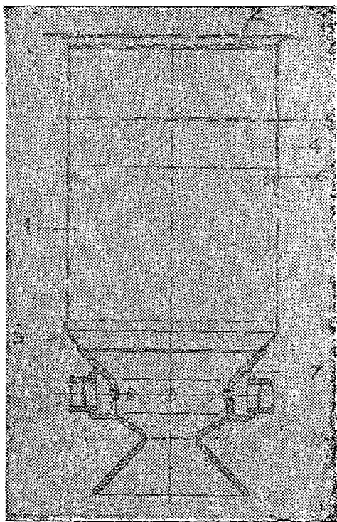
Рис. 12. Бункер газогенератора в сборе: 1—корпус бункера; 2—фланец бункера; 3—переходный конус бункера; 4—облицовка бункера; 5—отражатель газа; 6—крючки бункера; 7—камера газификации.
