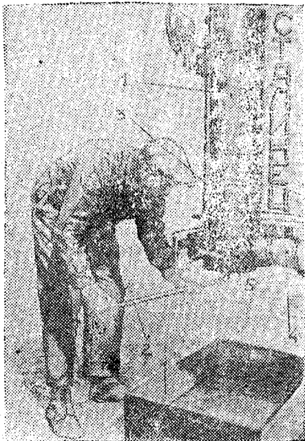
Рис. 37. Вывертывание опоры сеток колец Рашига в первом цилиндре фильтра: 1 -- цилиндры фильтра; 2 — ключ; 3 — карман подвода газа; 4 — патрубок подвода газа в фильтр; 5 — пробка люка.
