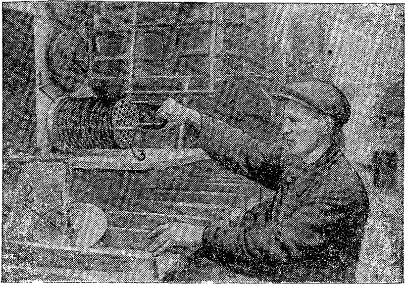
Рис 36. Разборка пластинчатого очистителя: 1—цилиндр пластинчатого очистителя; 2—крышки цилиндров; 3—секция.
