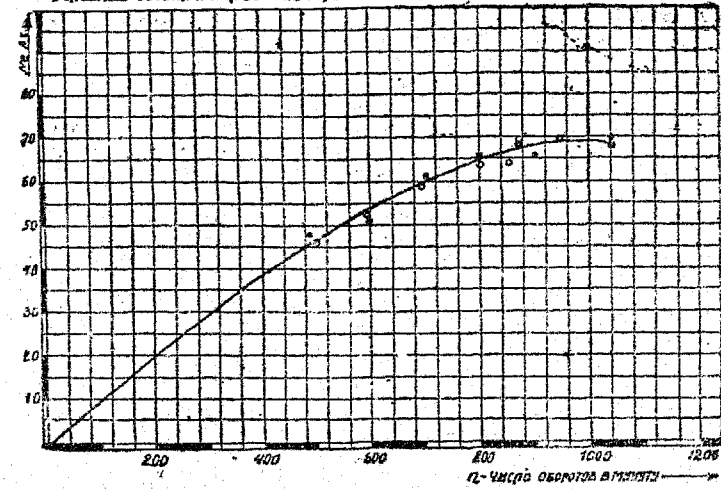
Рис. 42. Внешняя характеристика газового двигателя МГ-17 (топливо — березовые чурки).
