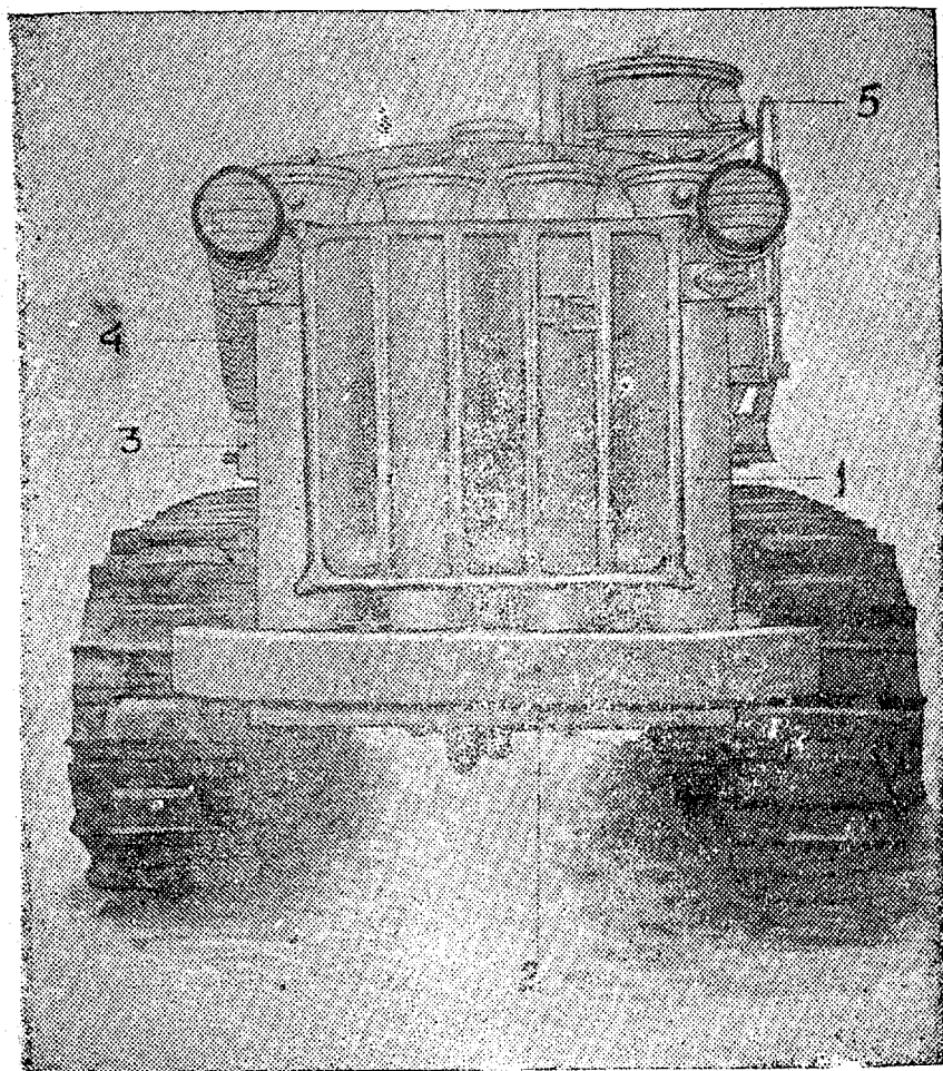
Рис. 7. Общий вид газогенераторной установки Г—25 на тракторе СТ—65 (вид спереди): 1—фильтр газа; 2—бампер; 3—отстойник; 4—соединительный шланг фильтра с отстойником; 5—газогенератор.
