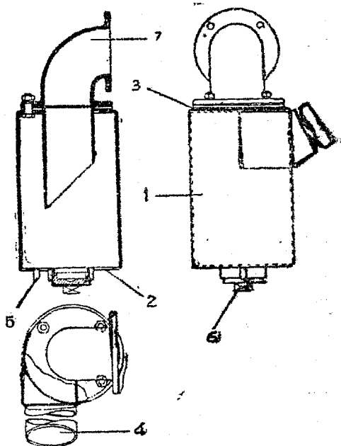
Рис. 19. Отстойник в сборе: 1—корпус; 2—дно корпуса; 3—крышка корпуса; 4—патрубок подвода газа; 5—сливная трубка; 6—пробка люка; 7—патрубок отвода газа.
