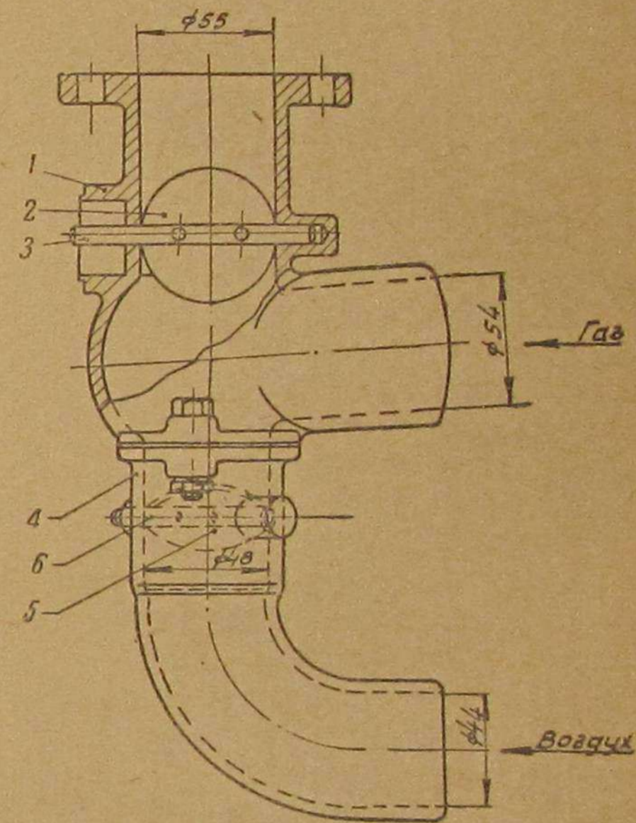
Фиг. 10. Смеситель.
