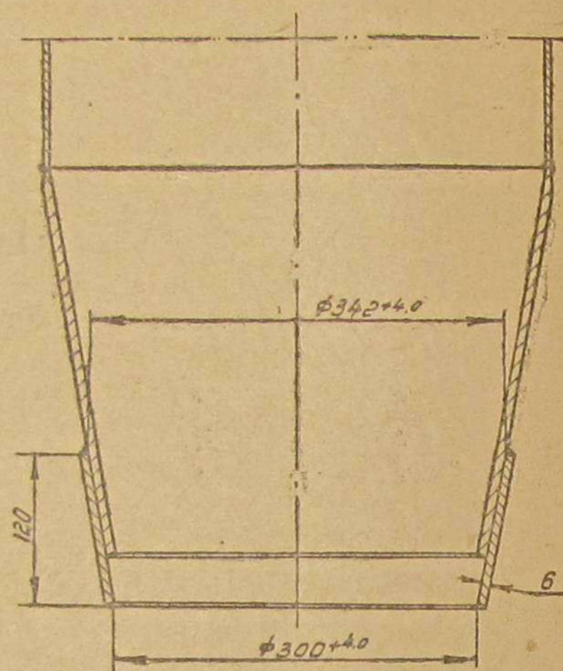
Фиг. 32. Эскиз для восстановления изношенного корпуса камеры газификации газогенератора Г58У-01А, предназначенного для газификации только древесных чурок.
