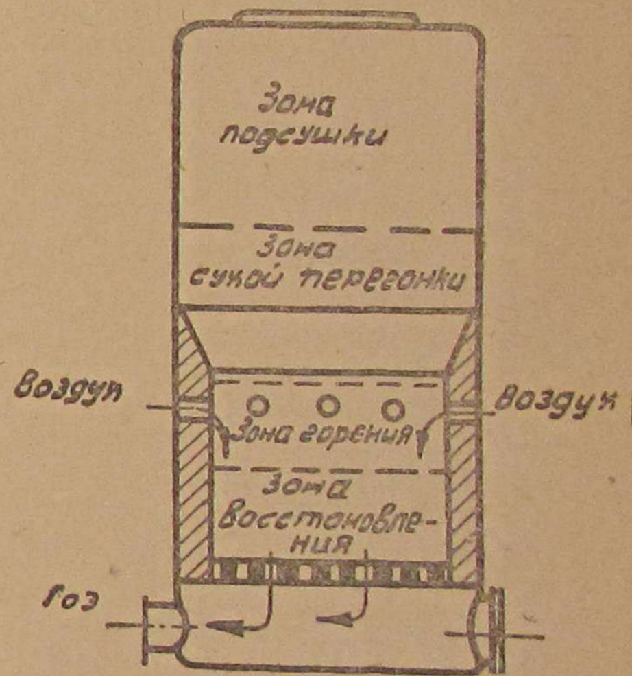
Фиг. 1. Схема газогенератора опрокинутого процесса.
