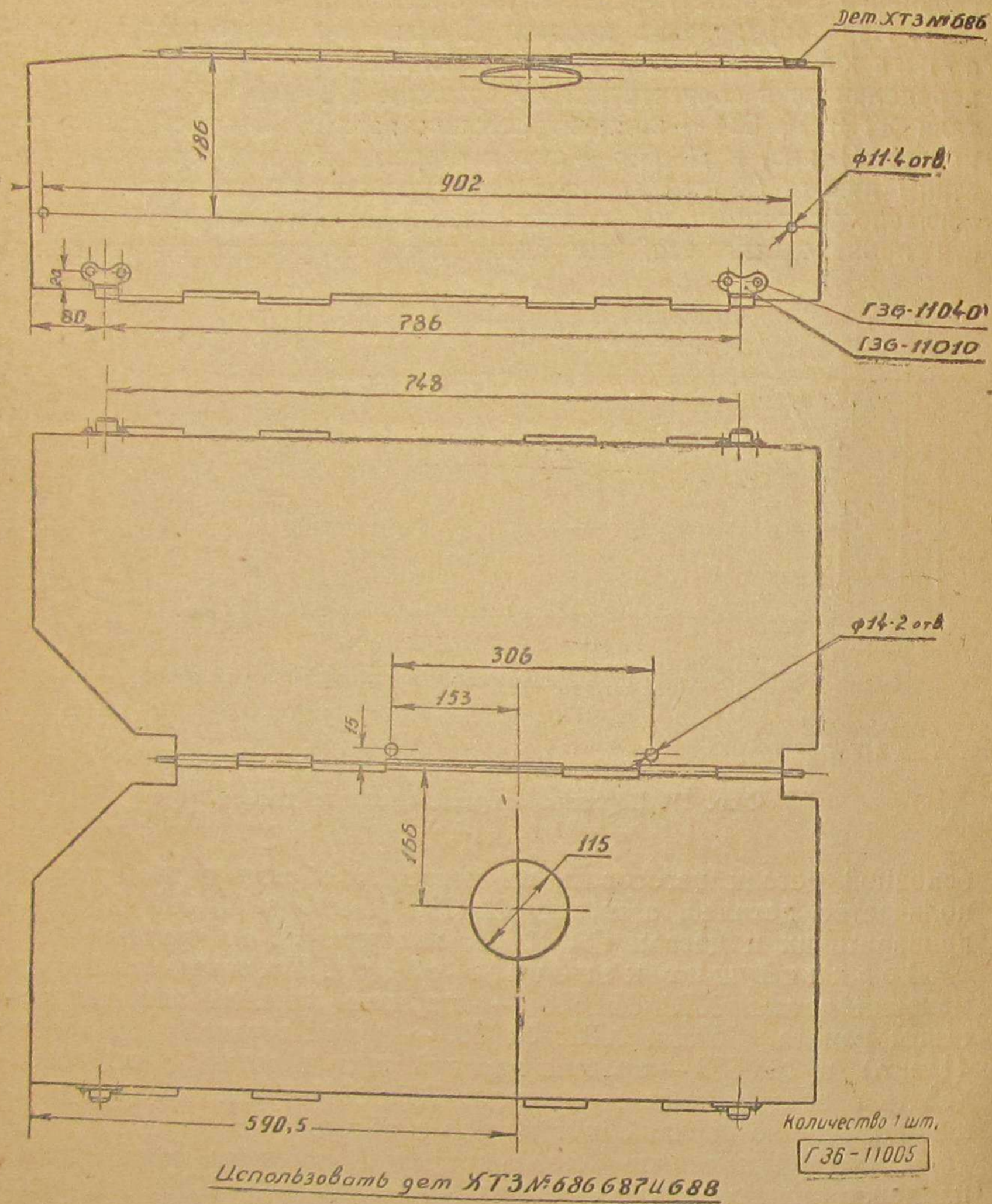
Фиг. 12. Верхний щит капота в сборе.
