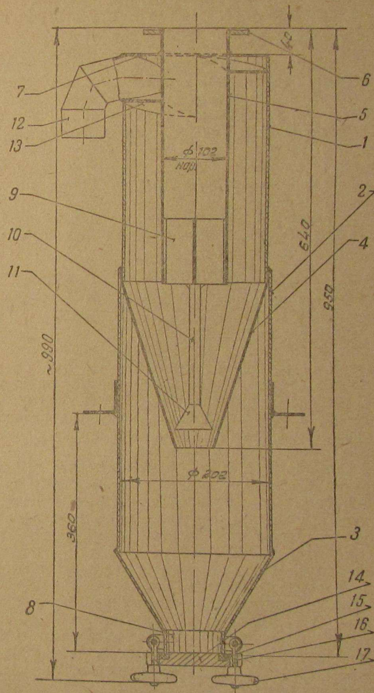
Фиг. 5. Циклон.
