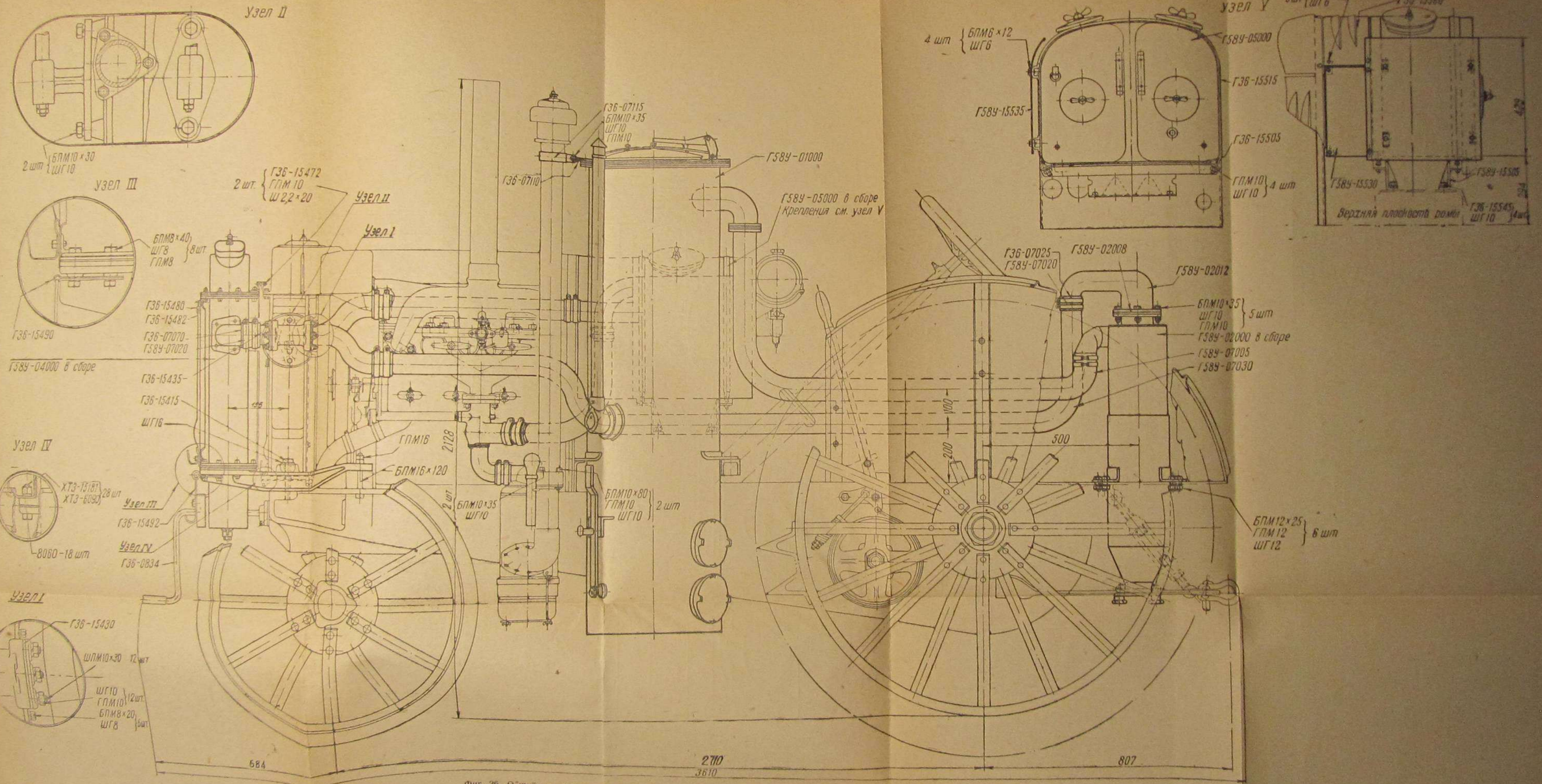
Фиг. 26. Общий вид газодвигательного трактора и крепление отдельных агрегатов газодвигательной установки (вид сбоку).
