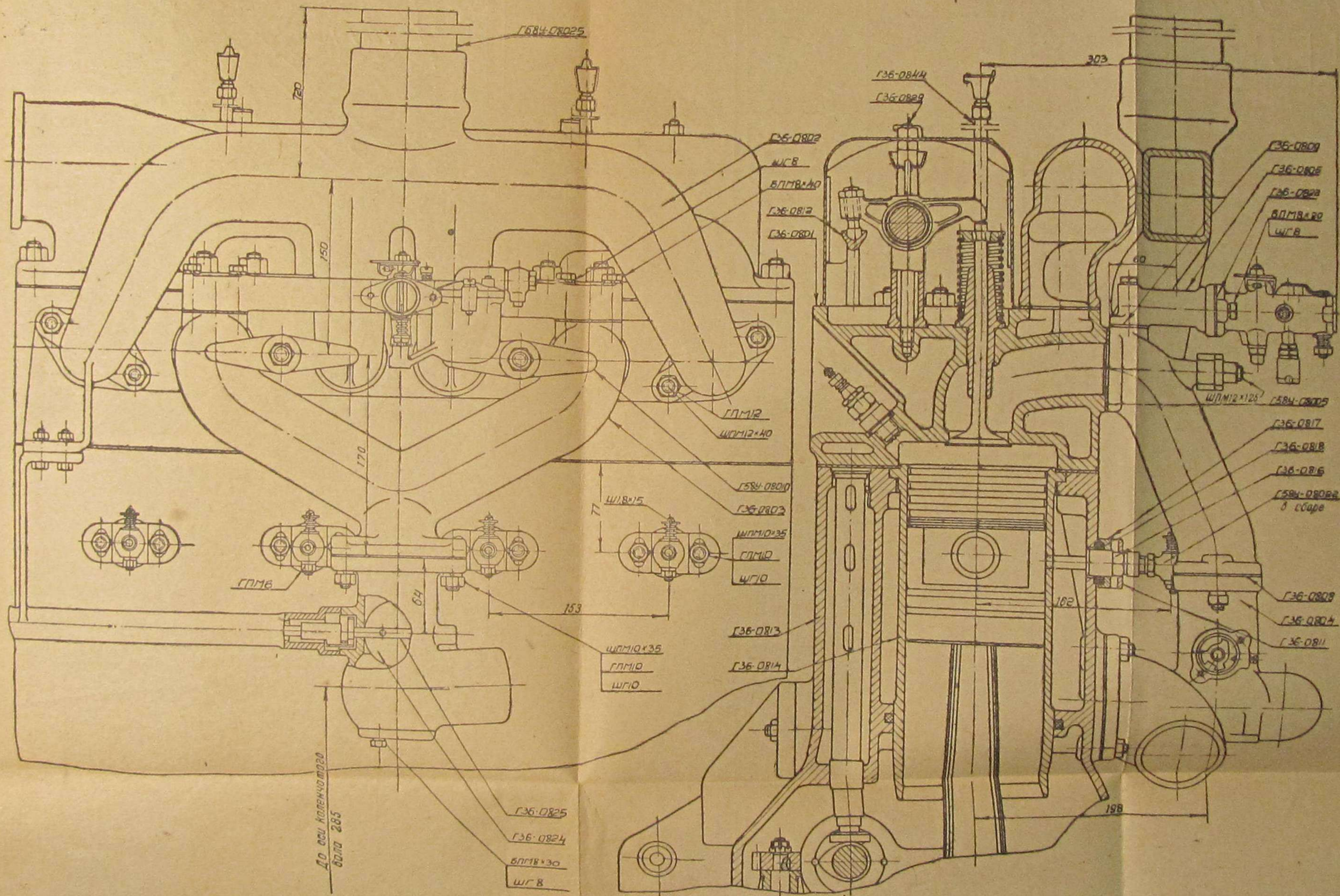
Фиг. 9. Общій вид газового двигателя СХТЗ-1Г.
