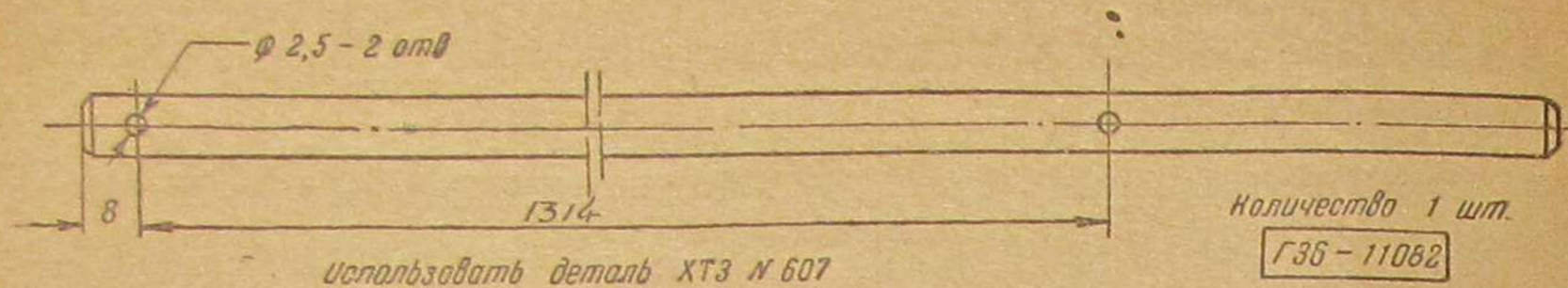
Фиг. 20. Ручная тяга дроссельного клапана.
