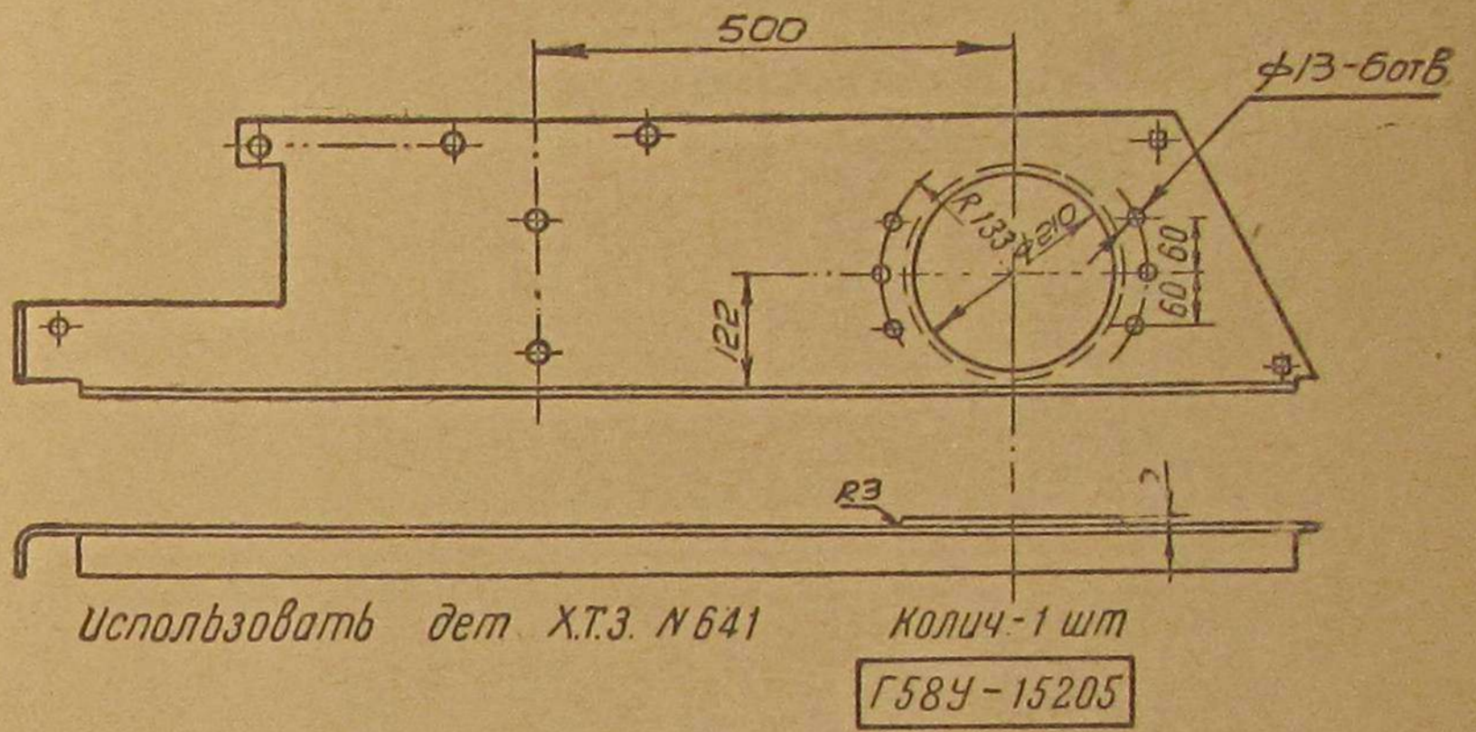
Фиг. 18. Левая пластина платформы.
