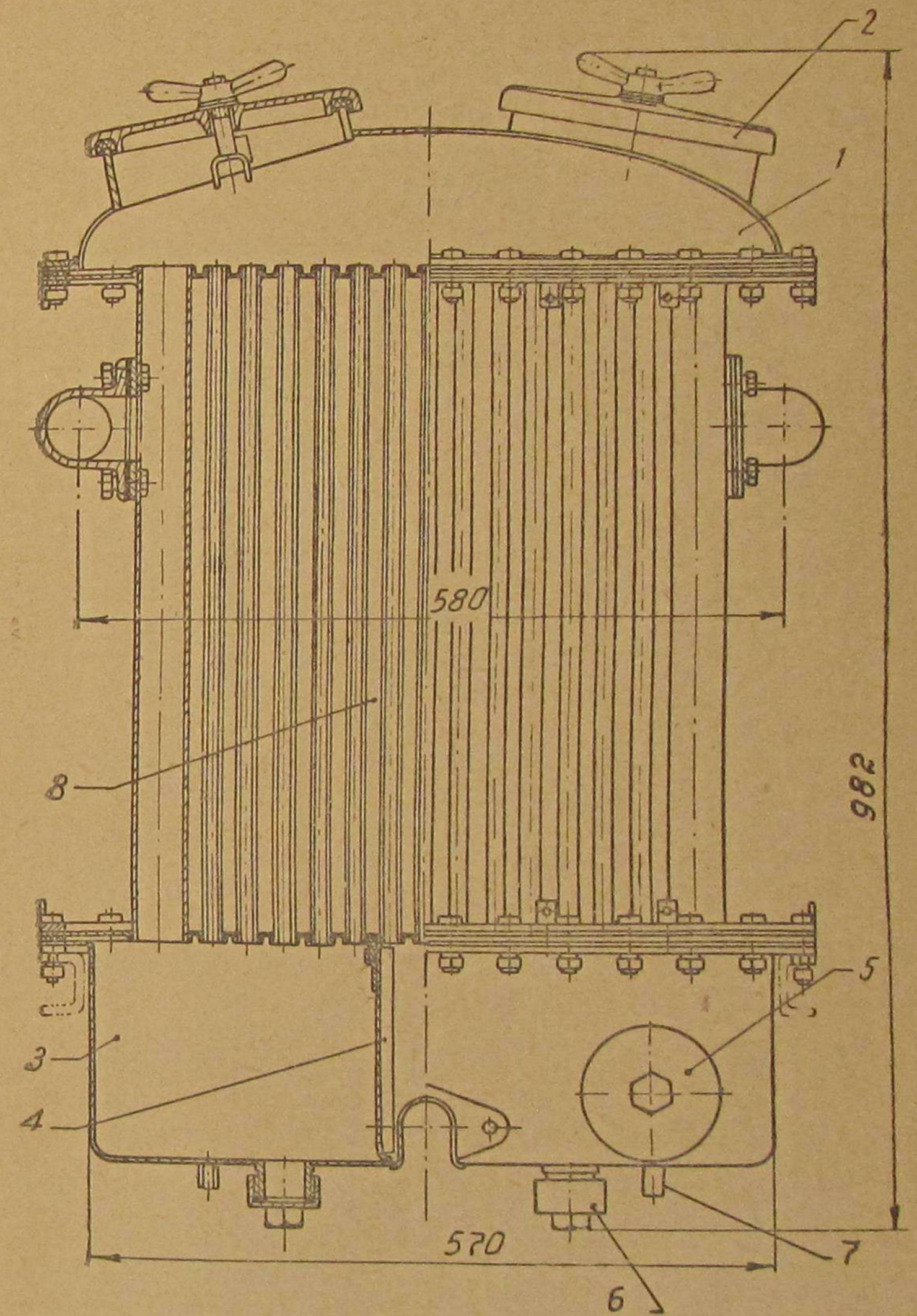
Фиг. 6. Охладитель.
