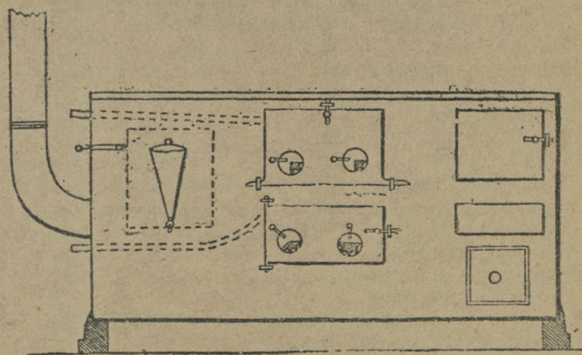
Рис. 33. Переносная печь.
