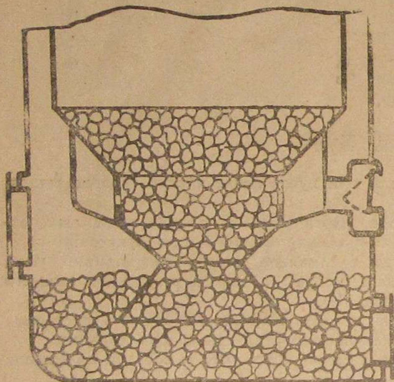
Фиг. 9. Уровень засыпки угля при загрузке.
