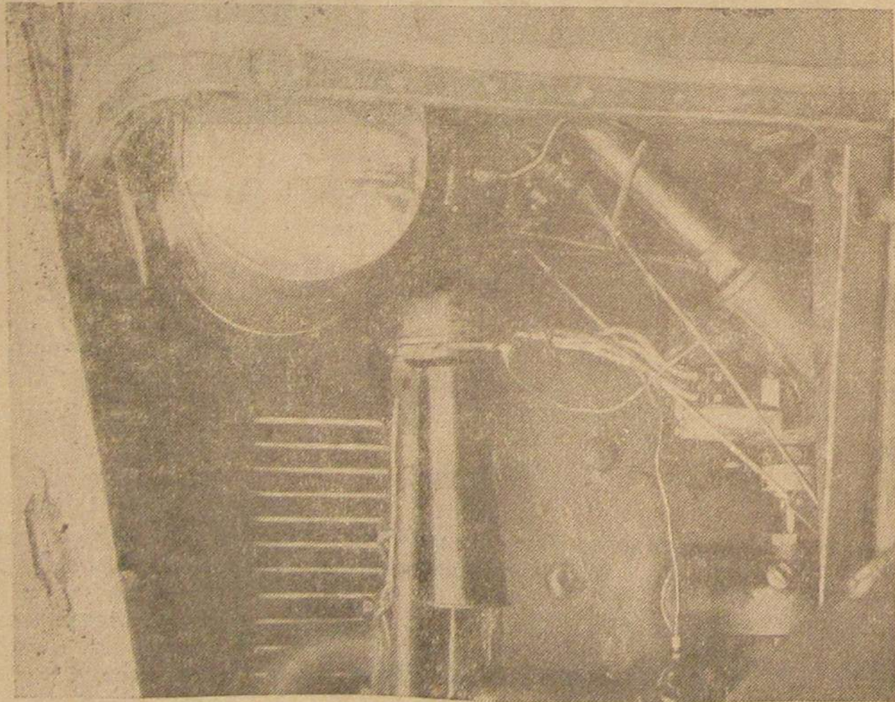
Фиг. 12. Вид на двигатель со стороны магнето. На щитке виден бензобачек и краник бензопровода.
