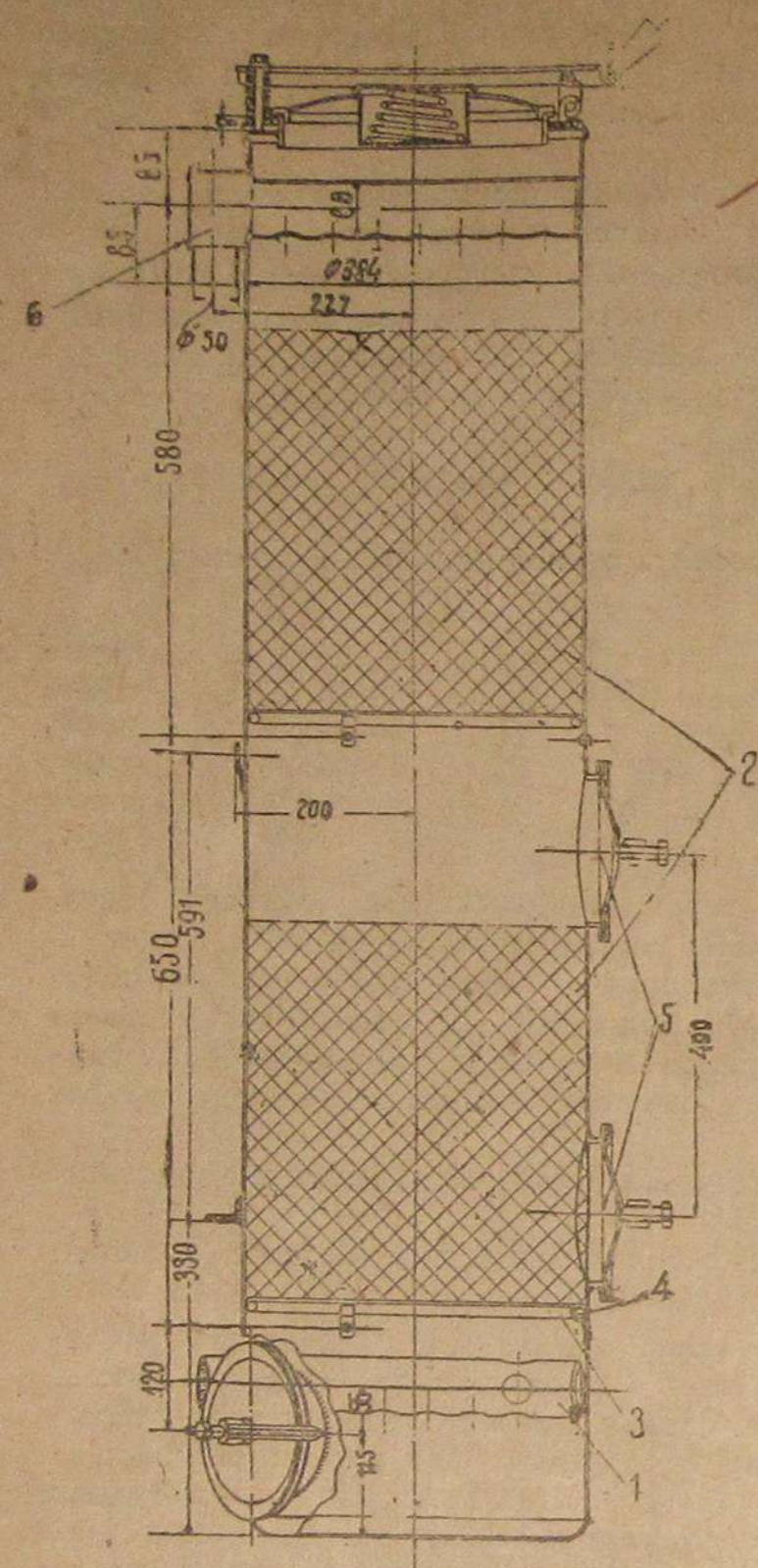
Фиг. 6. Вертикальный очиститель — ЗИС 13.
