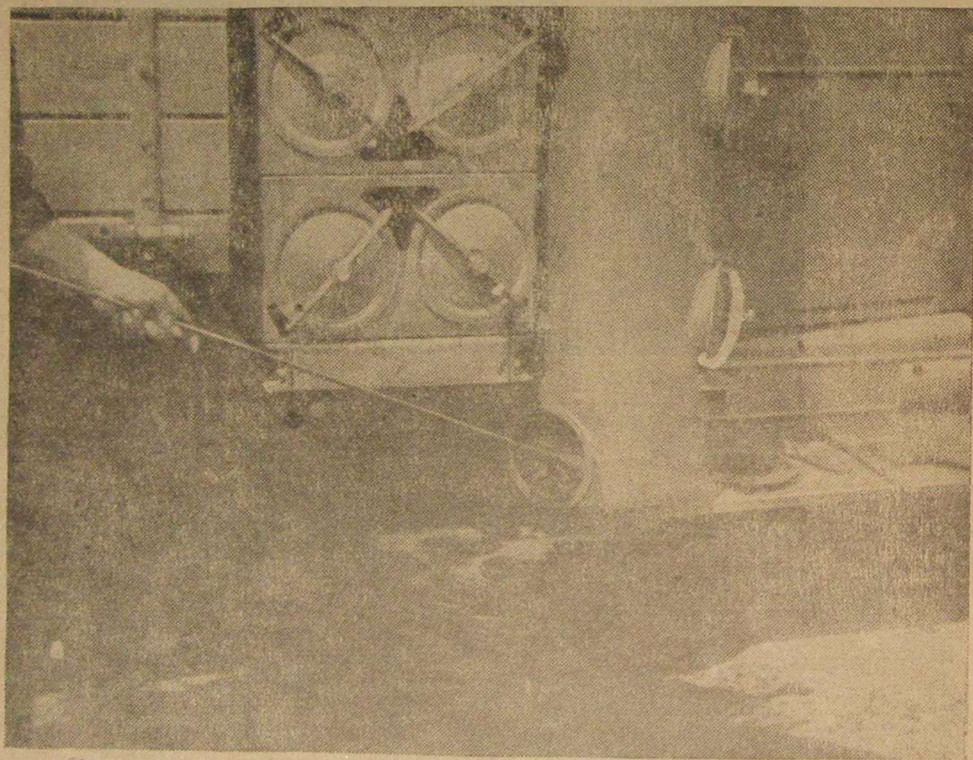
Фиг. 16. Чистка вертикального очистителя ЗИС-13.
