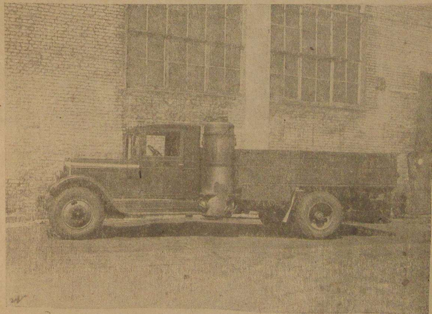
Фиг. 1. Общий вид автомобиля ЗИС—13 со стороны газогенератора.
