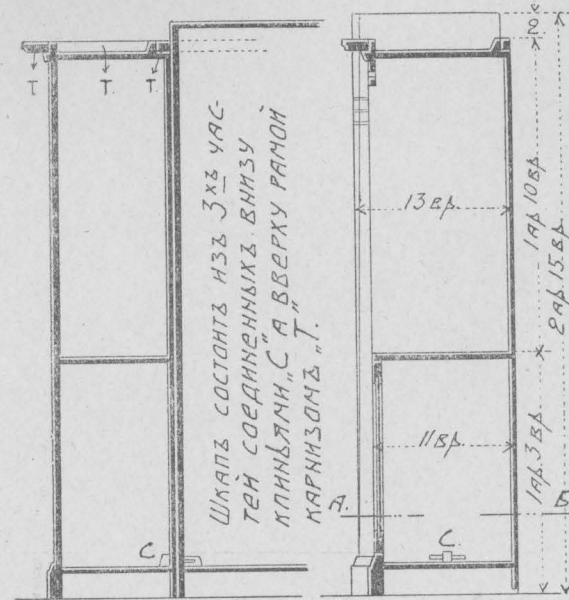
РАЗРѢЗЪ ПО А. Б.
