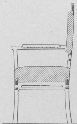
РАЗРЪЗЪ КРЕСЛА.
