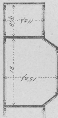
РАЗРЪЗЪ ПО ЛИНІИ В.Г.
