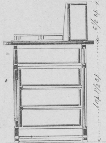
ВЕРТИКАЛЬНЫЙ РАЗР.
