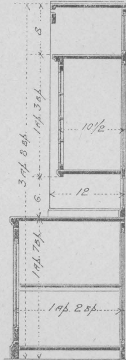
ВЕРТИКАЛЬН. РАЗР.
