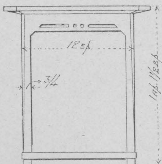
БОКОВОЙ ВИДЪ.
