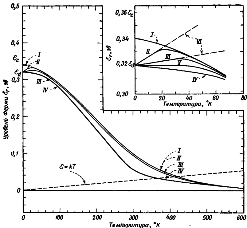
Фиг. 136. Зависимость положения уровня Ферми от температуры при различных концентрациях акцепторов. N_d = 10^{16} см ^{-3} .
