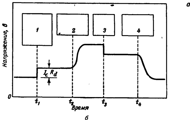
Фиг. 25. Опыт по исследованию движения дырок, введенных в германий p -типа.
