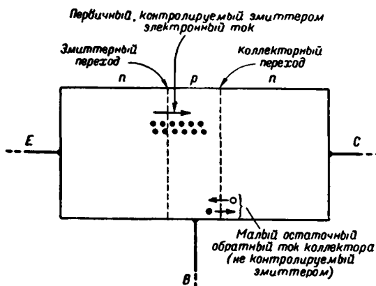
Ф и г. 3. Схема транзистора с n-p-n -переходами.
