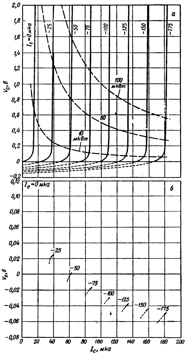
Ф и г. 6. Статические характеристики транзистора М 1752 для области более низких напряжений. а — для коллектора; б — для эмиттера.
