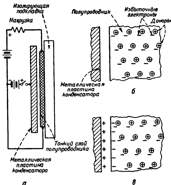
Фиг. 17. Модуляция проводимости 1 поверхностными зарядами.
