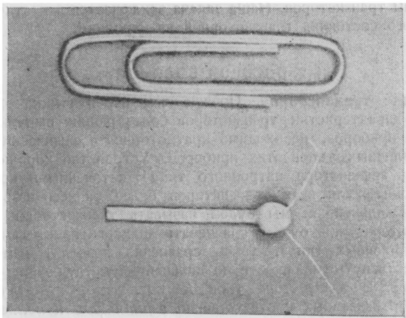
Фиг. 1. „Бусинковый“ транзистор (тип М 1689).
