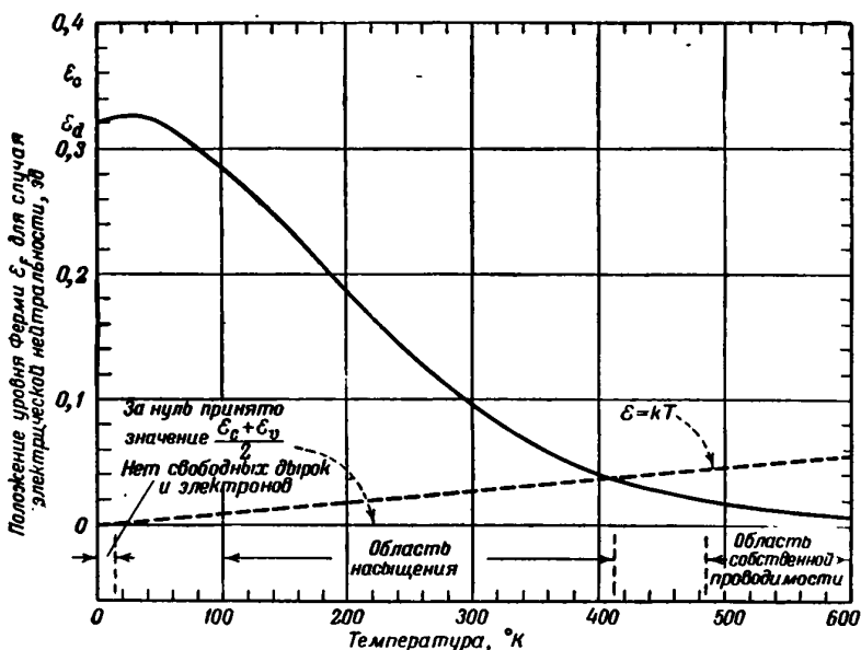
Ф и г. 92. Зависимость положения уровня Ферми от температуры для случая электрической нейтральности в образце германия с N_d = 10^{15} \text{ см}^{-3} , N_a = 10^{14} \text{ см}^{-3} и \mathcal{E}_v - \mathcal{E}_c = 0,04 \text{ эв} .
