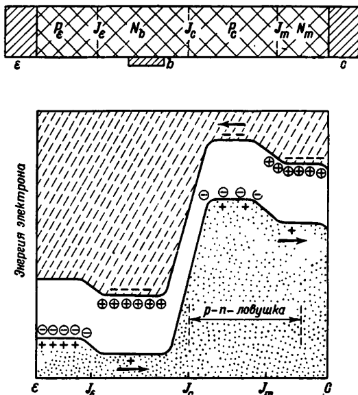
Фиг. 49. Транзистор с коллекторной областью усиления тока.
