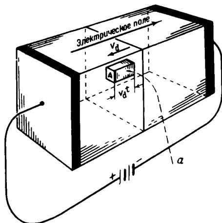
Ф и г. 79. Соотношение между скоростью дрейфа и током.
