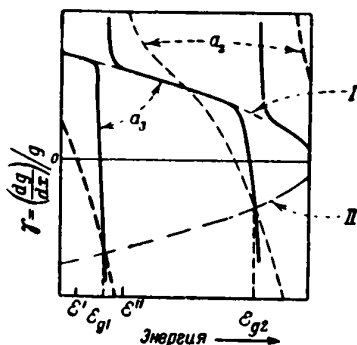
Фиг. 124. Зависимость \gamma от энергии на границе ямки ( x = a/2 ) (приближенно).
