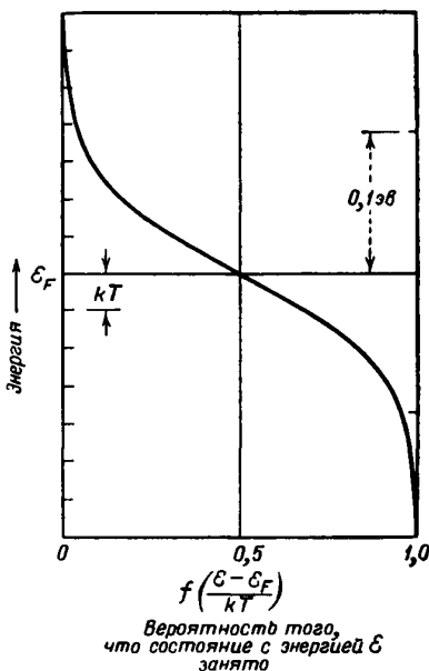
Фиг. 87. Функция распределения Ферми — Дирака.
