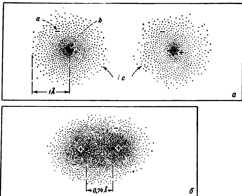
Фиг. 2. Парно-электронная связь в молекуле водорода. a — два атома водорода; б — молекула водорода.
