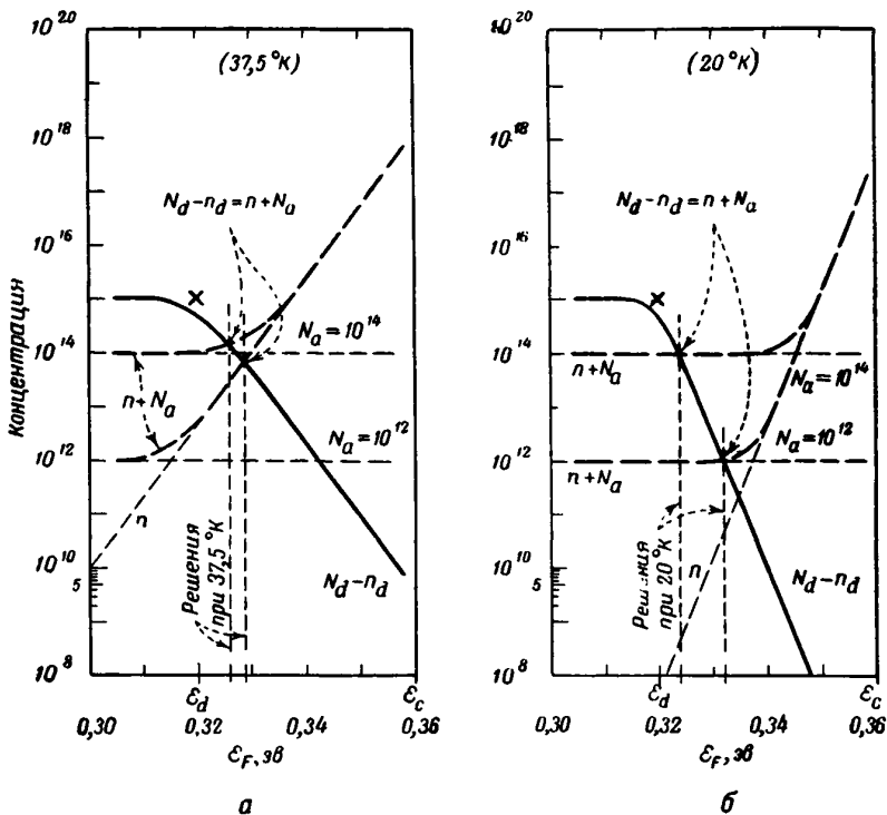
Фиг. 135. Значение \xi_F при N_a = 10^{14} \text{см}^{-3} и 10^{12} \text{см}^{-3} , N_d = 10^{15} \text{см}^{-3} , T \approx 37,5 и 20^\circ \text{К} .
