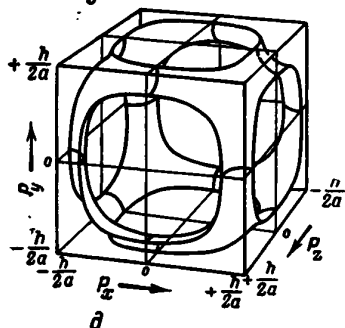
Фиг. 60. Зона Бриллюэна, разрешенные квантовые состояния и контуры равной энергии.
