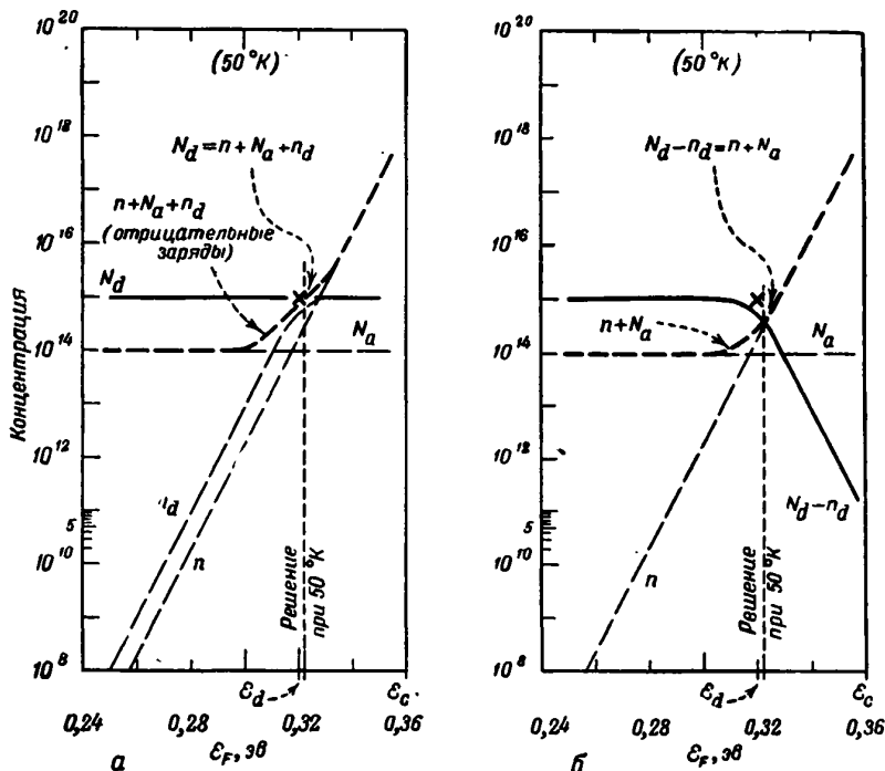
Фиг. 134. Значение \epsilon_F при N_a = 10^{14} см ^{-3} , N_d = 10^{15} см ^{-3} и T \approx 50^\circ\text{K} .
