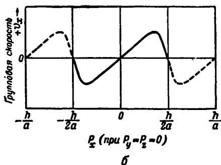
Фиг. 69. Энергия и скорость в зонах Бриллюэна. а — энергия как функция квази-импульса; б — групповая скорость для верхней энергетической зоны.
