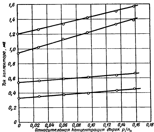
Ф и г. 30. Зависимость коллекторного тока I_c от среднего значения концентрации дырок, введенных в коллектор.
