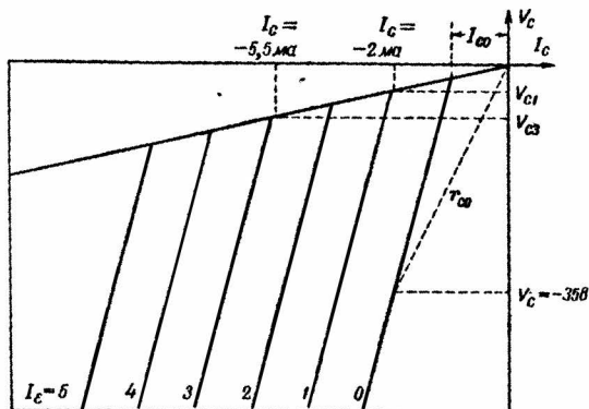
Фиг. 13. Идеализованные характеристики коллектора.
