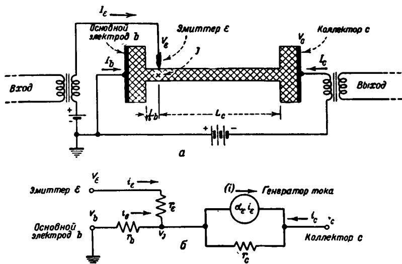
Фиг. 37. Нитевидный транзистор и его эквивалентная схема.
