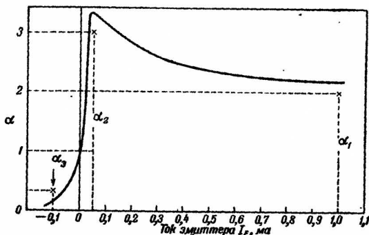
Фиг. 14. Зависимость эффективного значения коэффициента усиления по току \alpha от тока эмиттера.
