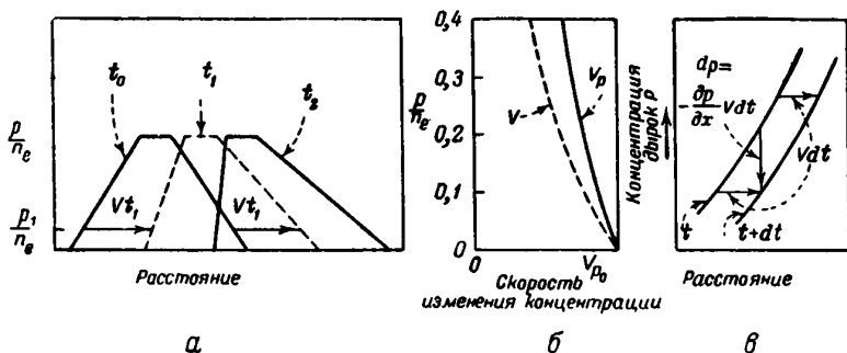
Фиг. 113. Деформация импульса дырочного тока, обусловленная модуляцией проводимости (для случая b=2 ).
