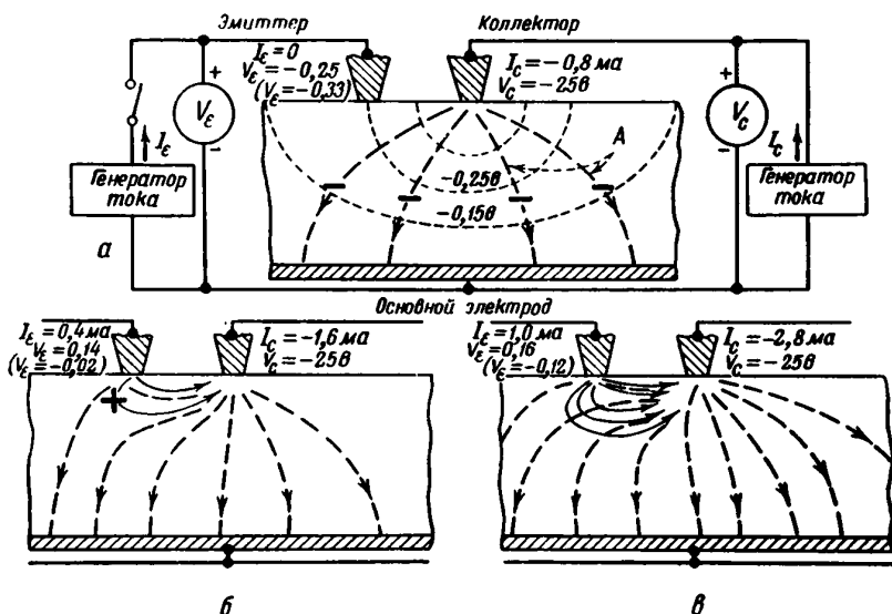
Фиг. 46. Диаграмма токов в транзисторе.
