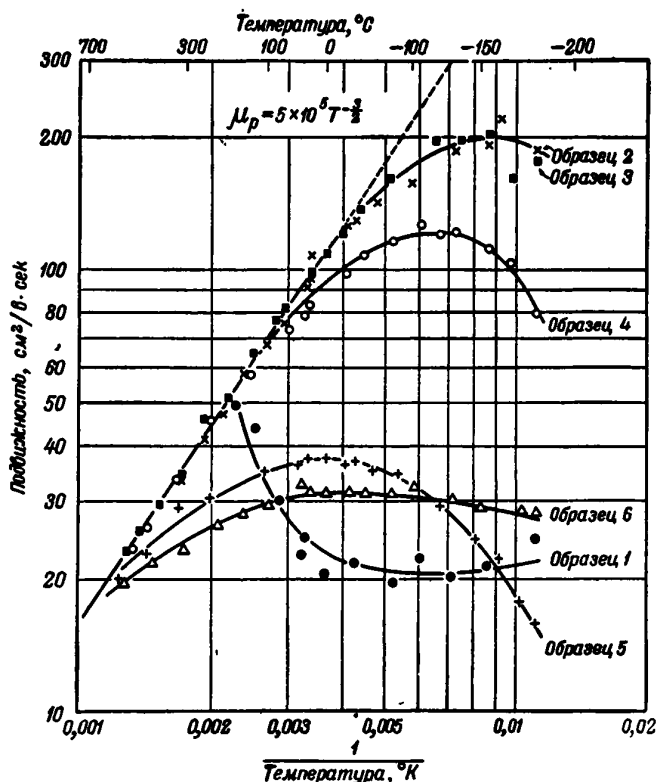
Фиг. 103. Зависимость подвижности дырок в сплавах кремния с бором от температуры.
