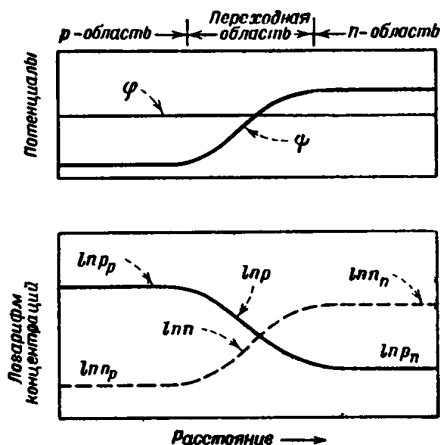
Фиг. 107. Зависимость n и p от потенциала \psi и положения уровня Ферми \varphi для p-n -перехода в случае более высокой проводимости в p -области.
