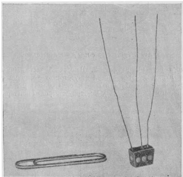
Фиг. 4. Внешний вид улучшенной модели транзистора с n-p-n -переходами (тип М 1752).
