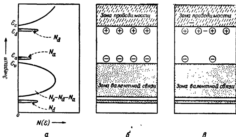
Фиг. 85. Схемы энергетических уровней.
