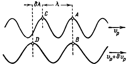
Фиг. 128. Сложение двух волн при образовании волнового пакета.
