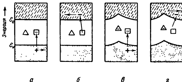
Ф и г. 118. Модуляция процесса рекомбинация — эмиссия захваченным зарядом.
