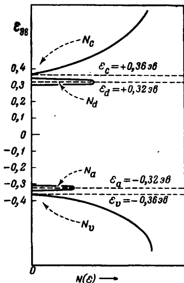
Ф и г. 130. Распределение квантовых состояний по энергиям.
