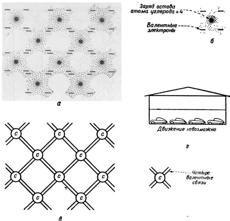
Фиг. 5. Электроны в структуре алмаза.
