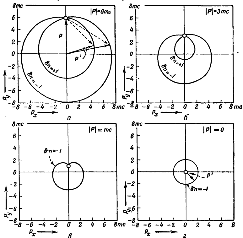
Фиг. 144. Начальные и конечные значения P для переходов, не сопровождающихся изменениями энергии.
