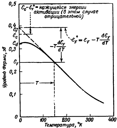
Фиг. 137. Кажущаяся энергия активации при N_a = 10^{14} \text{ см}^{-3} .
