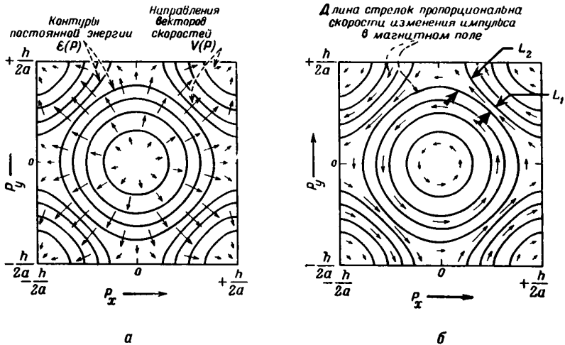
Фиг. 70. Влияние магнитного поля на энергию и скорость в зоне Бриллюэна. а — контуры равной энергии и распределение скоростей в плоскости P_z=0 ; б — изменение квази-импульса в магнитном поле, приложенном в направлении +z . \dot{\mathbf{P}} = -\frac{e}{c} \mathbf{V} \times \mathbf{H} (энергия максимальна в углах зоны).
