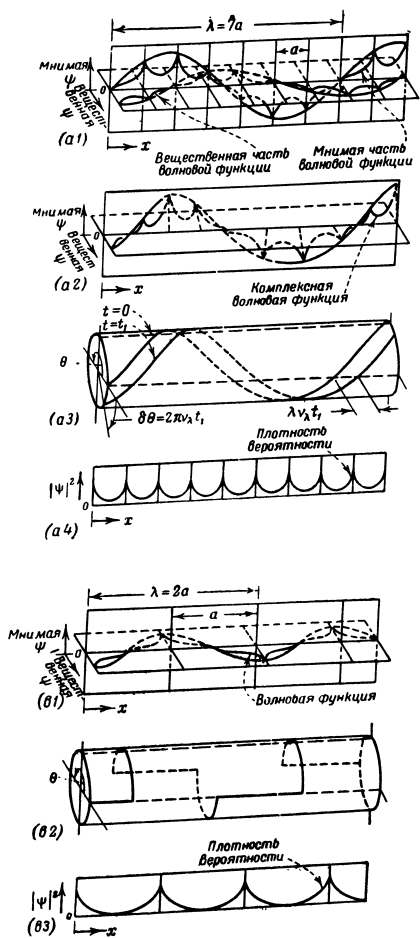
Фиг. 56. Волновая функция
