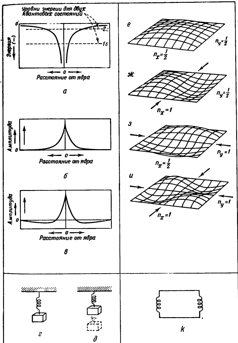
Фиг. 51. Волновые функции электрона и некоторые механические и электрические аналогии.
