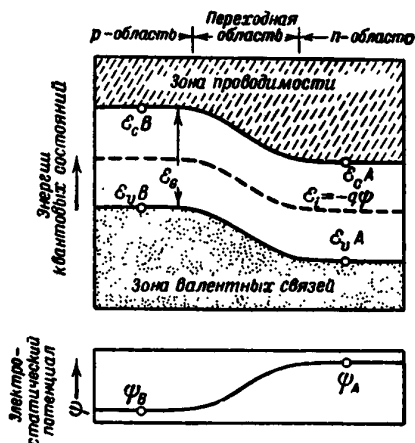
Ф и г. 106. Соотношение между уровнями энергии и электростатическим потенциалом.
