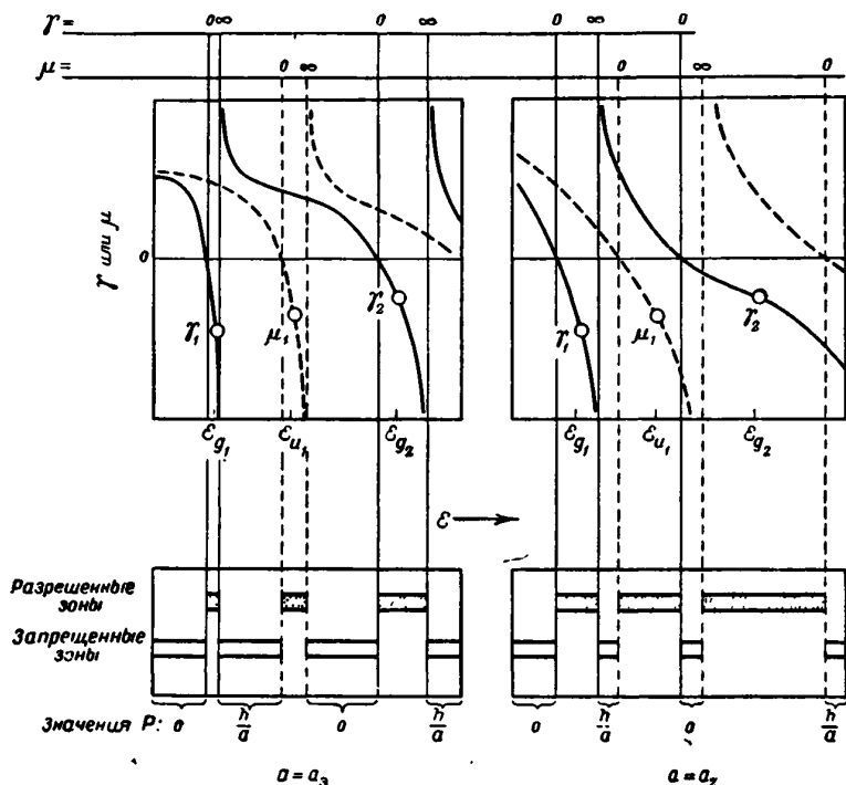
Фиг. 125. Структура энергетических зон при двух значениях постоянной решетки (приближенно).
