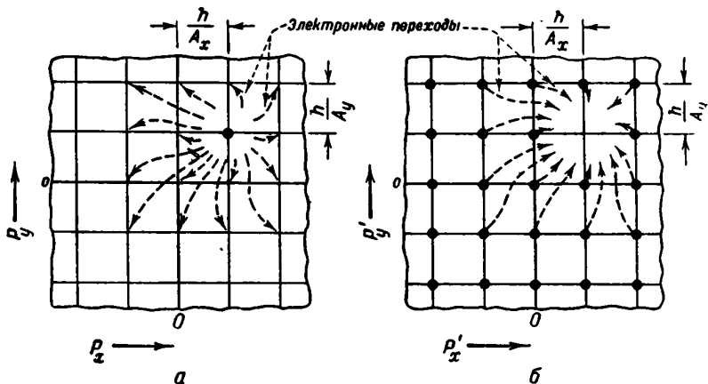
Фиг. 75. Возможные переходы для электрона и дырки.
