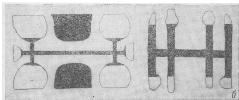
Фиг. 1. а — Микроманипулятор, использованный при исследовании движения введенных в германий дырок и электронов. б — Нитевидные образцы германия сложной формы с контактами большой площади. Длина левого образца 7,5 мм, правого — 3 мм.
