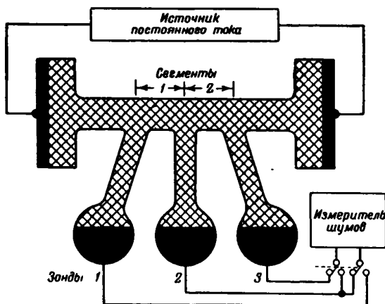
Фиг. 117. Схема опыта Монтегери для исследования шумов в германии.
