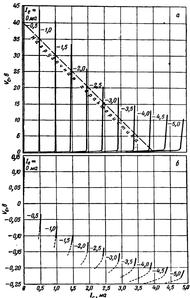
Ф и г. 5. Статические характеристики транзистора М 1752 с p-n-p -переходами.
