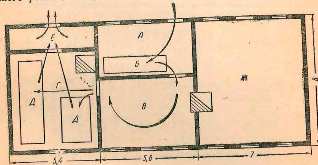
Рис. 111. План мастерской для выработки плетеных изделий: А — котельная, Б — котел, В — окорочный цех, Г — сушилка, Д — стеллажи, Е — буферный склад, Ж — цех для выработки плетеных изделий
