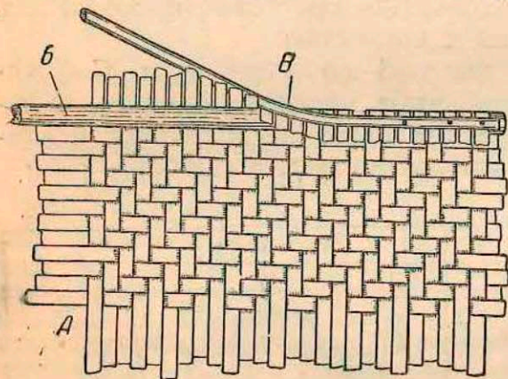
Рис. 87. Крепление полотна к рамке сиденья
