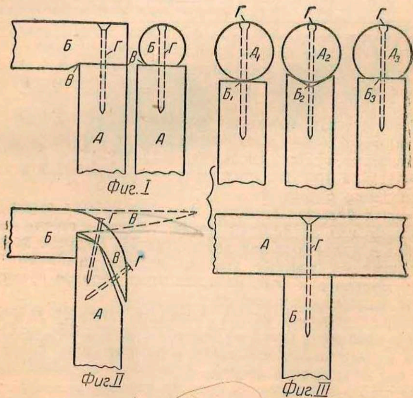
Рис. 72. Способы соединения деталей в плетеной мебели
