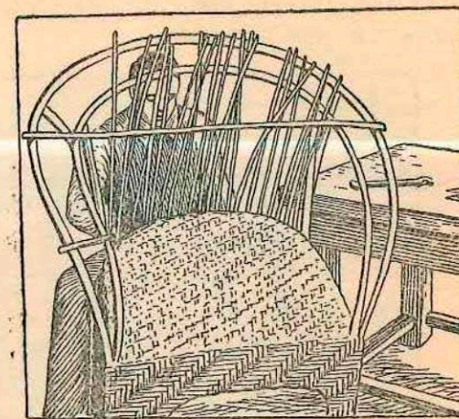
Рис. 90. Процесс установки дуг спинки и локотников
