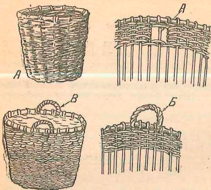
Рис. 54. Корзины плодовоовощные: верхние — с ручками-окошечками, нижние — с ручками-дужками
