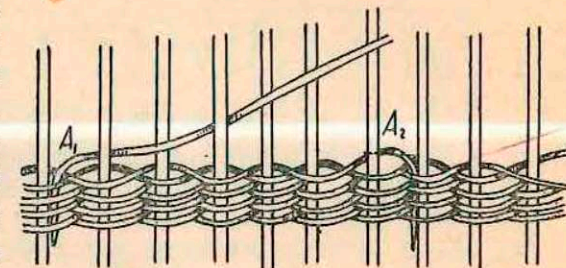
Рис. 47. Заделка концов прутьев утка внутрь плетеных стенок
