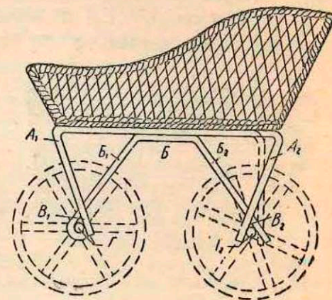
Рис. 62. Палочный ход под корзину детской коляски
