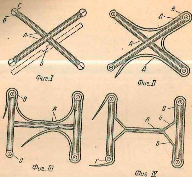
Рис. 75. Основные виды соединения ножек с проножками
