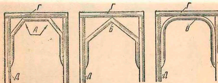
Рис. 73. Виды крепления подстрелок
