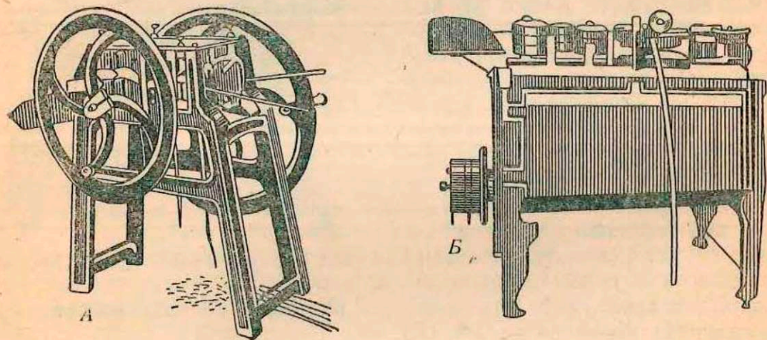
Рис. 20. Окорочные машины с цилиндрами: А — с ручным приводом, Б — со шкивом для работы от двигателя
