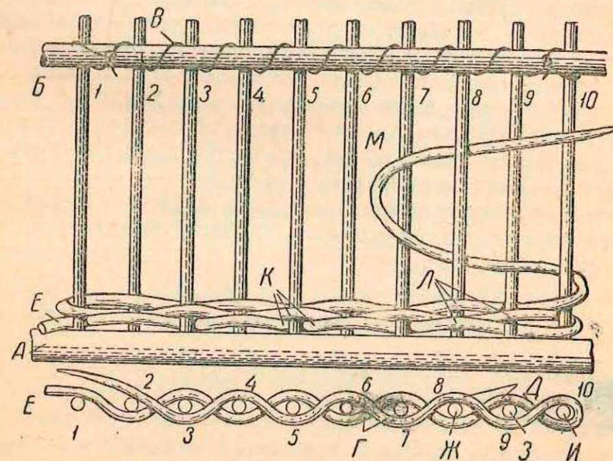
Рис. 36. Схема простого плетения
