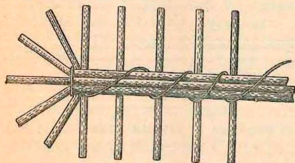
Рис. 35. Основа для плетения овального щитка
