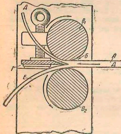
Рис. 30. Схема строжки лент на станке «шиф»
