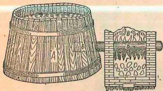
Рис. 18. Приспособление деревянного бака для проварки прута
