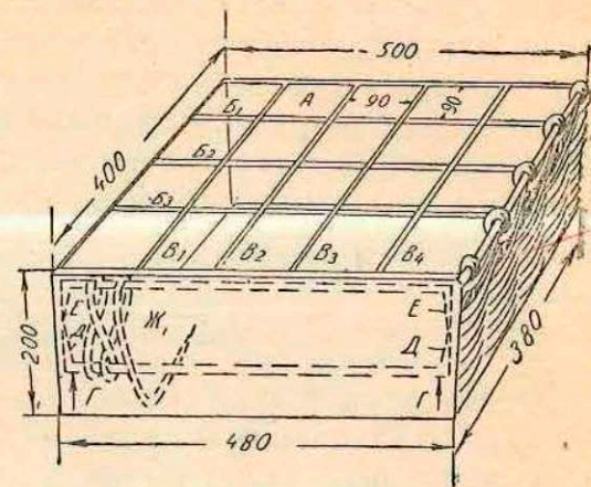
Рис. 58. Корзина для пивных бутылок (размеры в мм)
