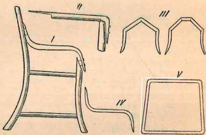
Рис. 84а. Детали остова кресла
