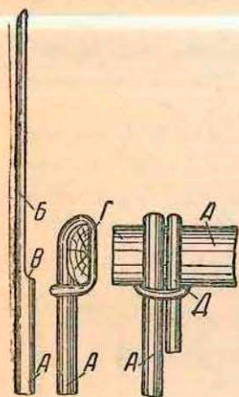
Рис. 32. Крепление прутяных стоек затяжной петлей
