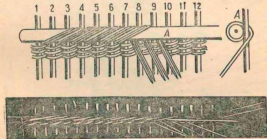
Рис. 45. Плетение толстого рядка
