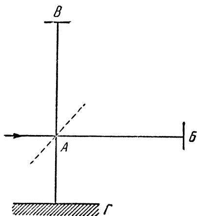
Рис. 2. Схема опыта Майкельсона. Полуперебрающее зеркало A разделяет световой луч. Одна часть идет вдоль движения Земли и отражается от B , другая — перпендикулярно движению Земли и отражается от B . С помощью A оба луча посылаются на экран Г для наблюдения интерференции. Если повернуть весь прибор на 45^\circ , оба луча оказываются в одинаковом положении относительно направления движения Земли.
