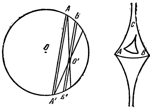
Рис. 9. Две модели плоскости Лобачевского. Слева наблюдатель, стоящий в точке O на равнине, видит две дороги: AA' и BB' . Линию горизонта он принимает бесконечно удаленной. Тогда из точки O' можно провести целый пучок прямых, нигде не пересекающих AA' в поле зрения O . Справа — тело вращения, на поверхности которого действует геометрия Лобачевского. Сумма углов треугольника ABC меньше 180^\circ .
