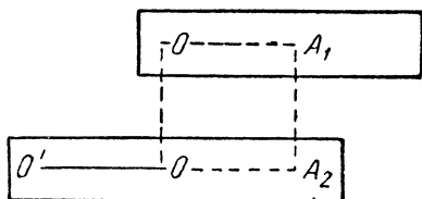
Рис. 4. Вывод закона сложения скоростей. Если отрезки OA_1 и O'A равны и время от послыски до приема сигнала одинаково и равно одной секунде, то скорость света относительно верхней системы отсчета численно равна отрезку OA_1 , а относительно нижней системы — отрезку O'A_2 .
