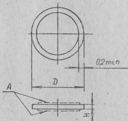
A — серебряная контактная поверхность
