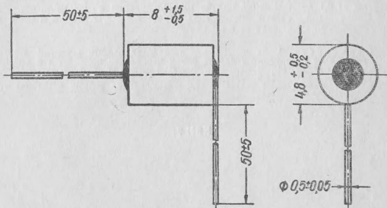
КВИ-2-15-22 пф
