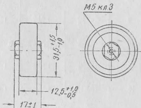
КВИ-3-12-1000 пф
