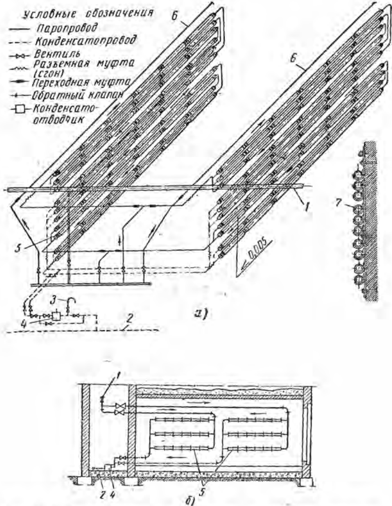
Рис. 37. Устройство сборных калориферов из чугунных ребристых труб в лесосушильных камерах с побудительной циркуляцией:
