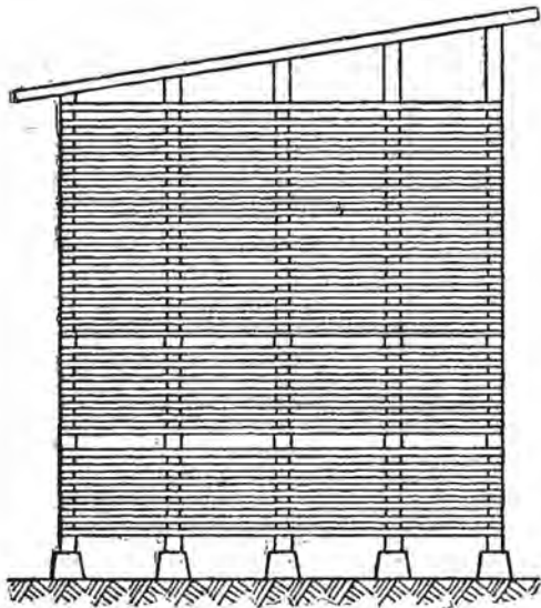
Рис. 100. Расположение горизонтальных каналов по высоте штабеля
