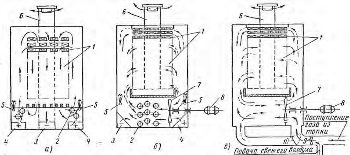
Рис. 13. Схемы устройства лесосушильных камер:
