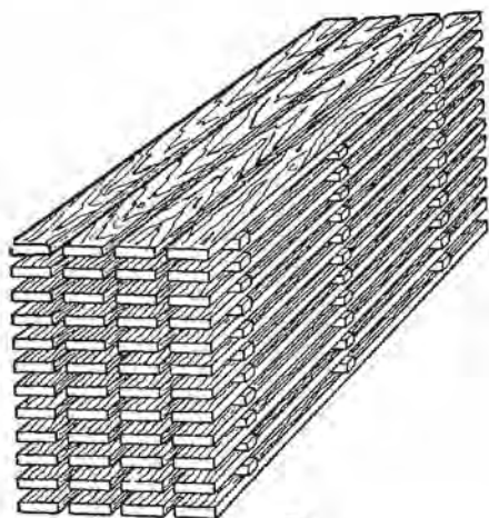
Рис. 96. Правильно (а) и неправильно (б) уложенный пакет
