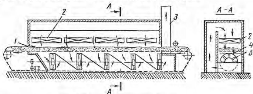
Рис. 114. Схема одноленточной сушилки:
