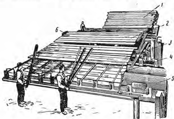
Рис. 69. Штабелеукладчик с ручной раскладкой прокладок:
