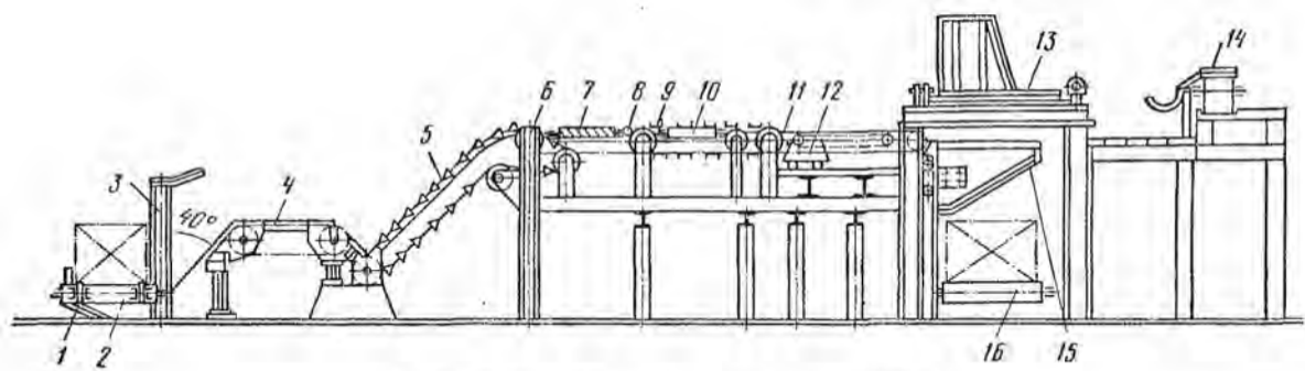
Рис. 70. Пакетоформирующая машина ПФМ-10:
