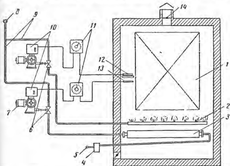
Рис. 63. Схема автоматического регулирования температуры и влажности сушильного агента с помощью ЭРА двух одноканальных регуляторов ЭРА:
