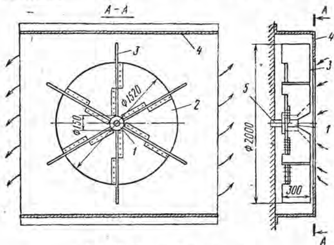
Рис. 45. Роторный вентилятор:
