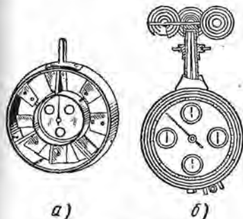
Рис. 64. Анемометры: а — крыльчатый, б — чашечный
