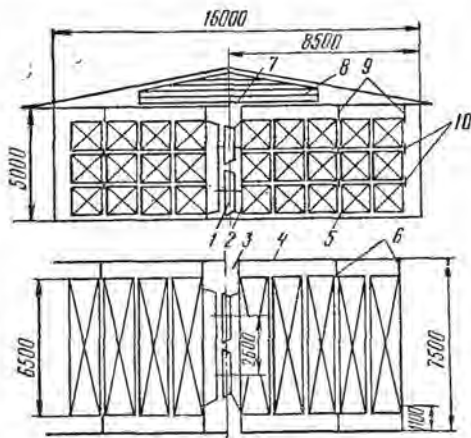
Рис. 107. Схема вентиляторной установки периодического действия ЦНИИМОД: 1 — вентилятор, 2 — упорная стенка с растробом, 3 — разрыв в боковой стенке, 4 — боковая стенка, 5 — пакет пиломатериала, 6 — боковые экраны, 7 — разрыв в потолке, 8 — жалюзийная решетка, 9 — потолочные экраны, 10 — щитки
