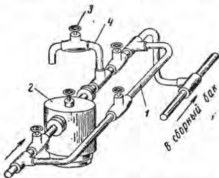
Рис. 40. Установка конденсатоотводчика:
