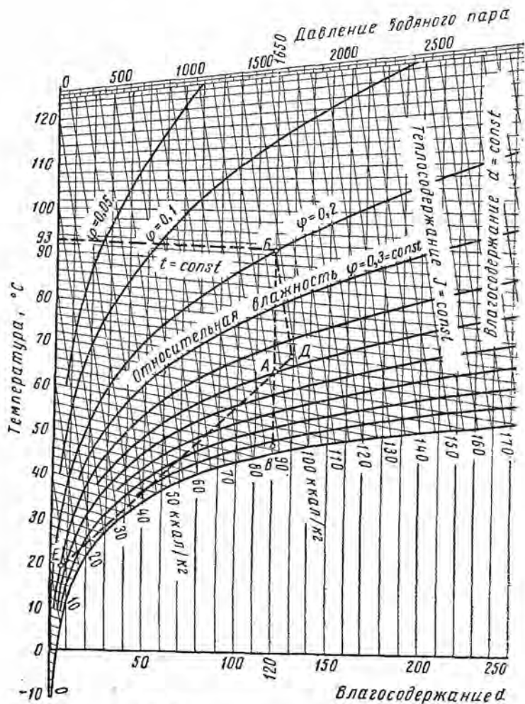
Рис. 2. t - d -диаграмма влажного воздуха
