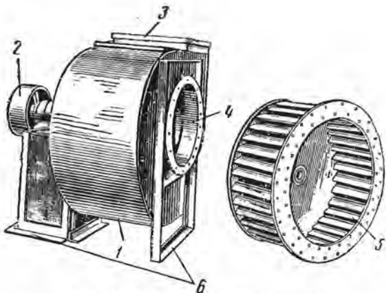
Рис. 44. Центробежный вентилятор:
