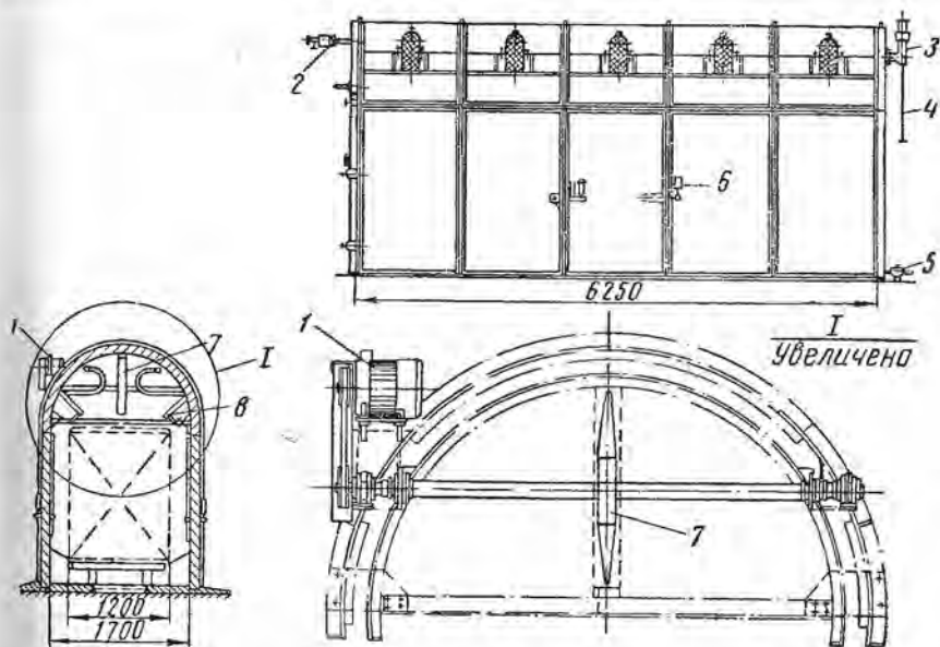
Рис. 25. Сборная металлическая сушильная камера Валмет (Финляндия): 1 — электродвигатели, 2 — ввод пара, 3 — выхлопная труба, 4 — тяга задвижки от выхлопной трубы, 5 — конденсатоотводчик, 6 — психрометр, 7 — вентилятор, 8 — калорифер
