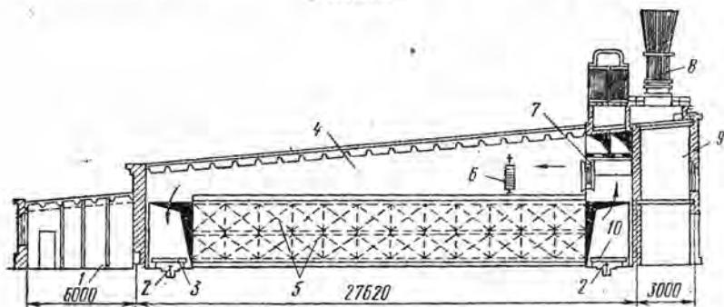
Рис. 31. Низкотемпературная лесосушильная камера для экспортных пиломатериалов (Гипродрев):
