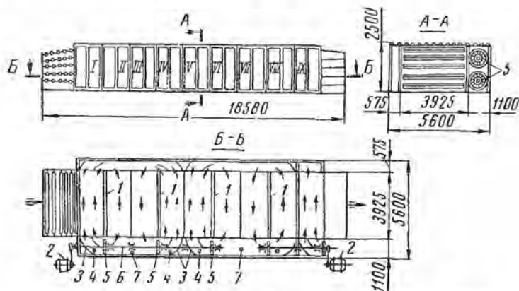
Рис. 110. Схема паровой сушилки СVP-4 с поперечной циркуляцией:
