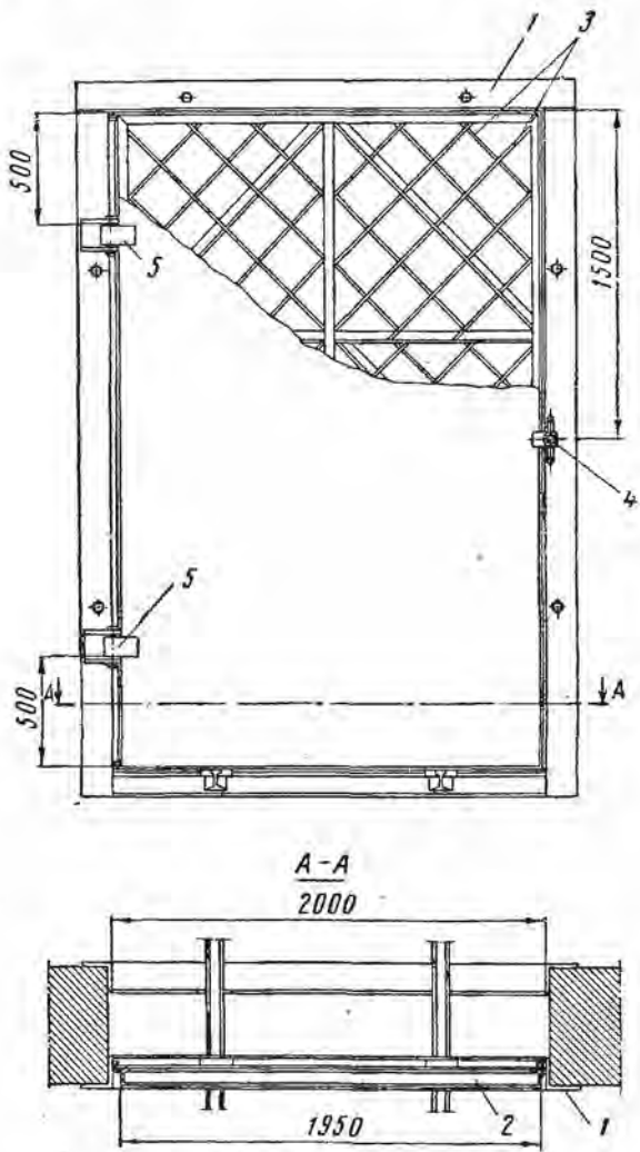
Рис. 35. Одностворчатая дверь: 1 — закладная рама, 2 — дверное полотно, 3 — решетка, заполненная утепляющим материалом, 4 — винтовой запор, 5 — дверная петля
