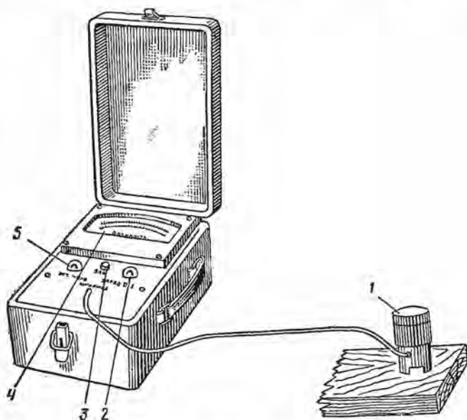
Рис. 7. Общий вид электровлагомера ЭВА-2М:
