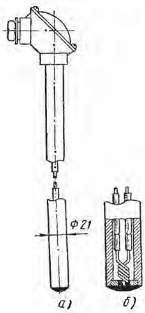
Рис. 60. Термопара ТХК-146:
