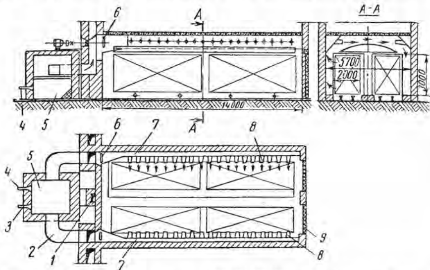
Рис. 23. Газовая сушильная камера ВНИИДМАШ — Моспроектстройиндустрия:
