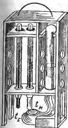
Рис. 55. Переносной психрометр
