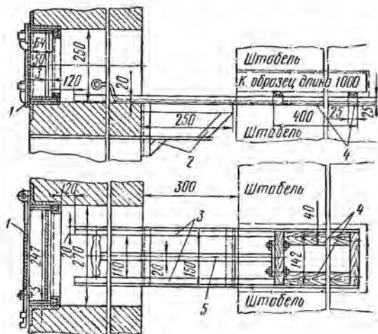
Рис. 122. Схема устройства приспособления для закладки образцов в камеры:
