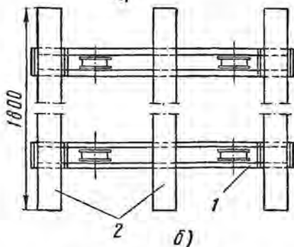
Рис. 75. Устройство трека и трековой тележки:
