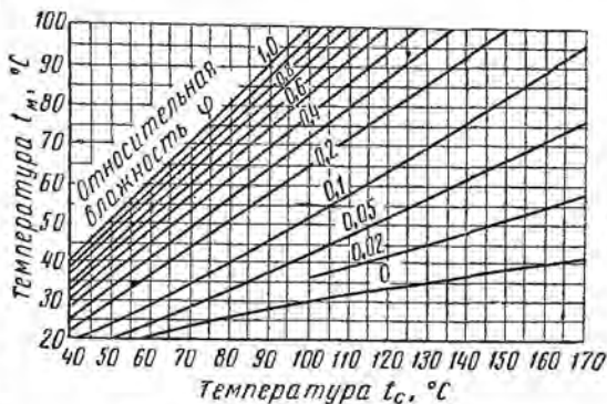
Рис. 1. Психрометрическая диаграмма
