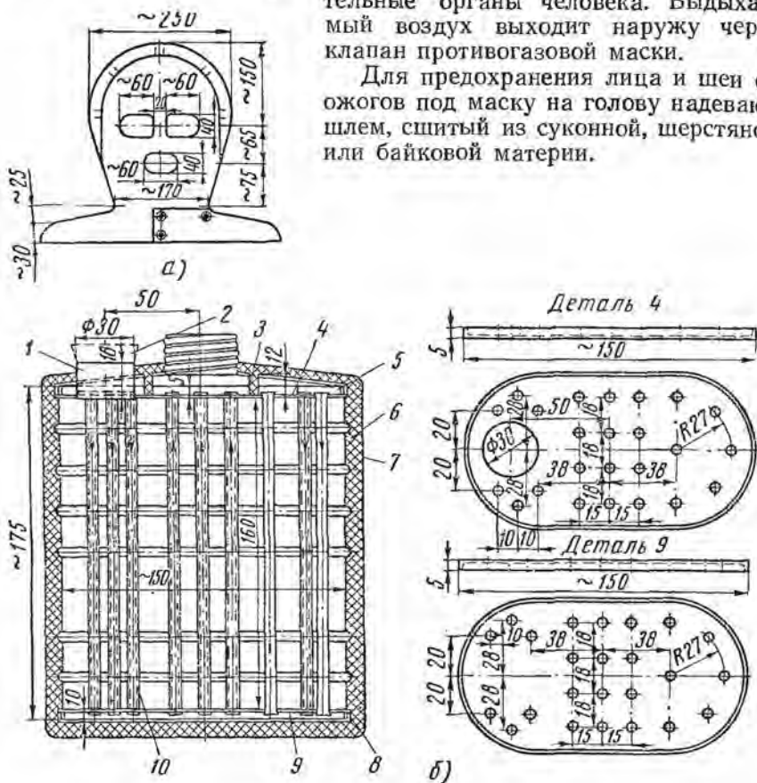
Рис. 124. Шлем (а) и охлаждающая коробка (б):
