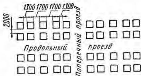
Рис. 93. Примерная планировка группы рядовых штабелей
