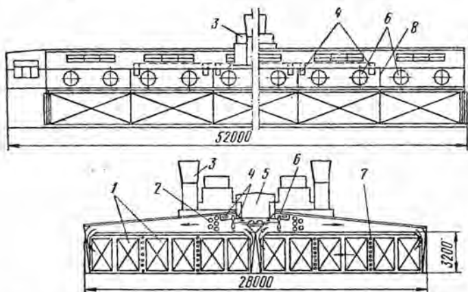
Рис. 30. Блок из двух сборных низкотемпературных сушильных камер ЦНИИМОД — ЛТА-65 непрерывного действия с поперечной циркуляцией воздуха и продольной загрузкой штабелей:
