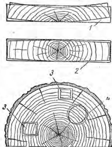
Рис. 8. Изменение формы поперечного сечения досок и деталей при усушке:
