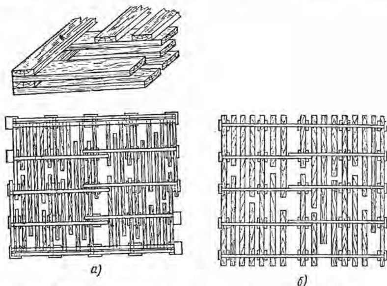
Рис. 98. Укладка пиломатериалов в рядовой штабель глубоким потем (а) и в рядовой штабель с выступающими концами (б)
