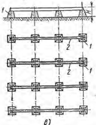
Рис. 95. Устройство штабельного фундамента из переносных элементов: a — бетонные опоры, б — деревянные опоры, в — общий вид фундамента; 1 — опора, 2 — балка, H — высота фундамента
