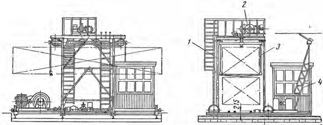
Рис. 71. Электрифицированная траверсная тележка ЭТ-20-II, оборудованная порталным подъемником:
