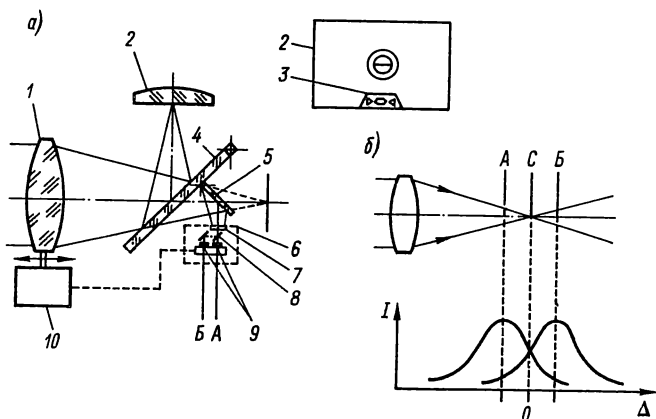
Рис 47. Схема автофокусировочной системы фотоаппарата «Пентакс МЭ-Ф» (а) и форма сигналов от двух линеек фотоприемников А и В (б):
