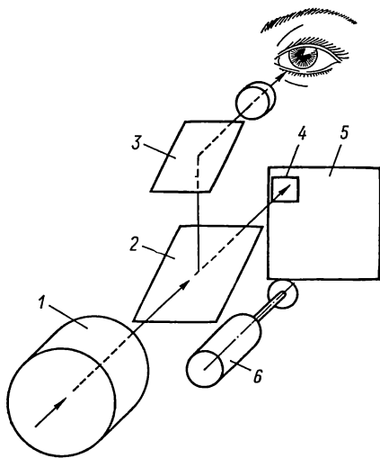
Рис. 58. Схема фотоаппарата с магнитной записью изображения
