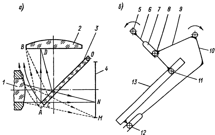
Рис. 30. Поворотное зеркало: a — схема движения зеркала обычной длины; b — привод удлиненного зеркала
