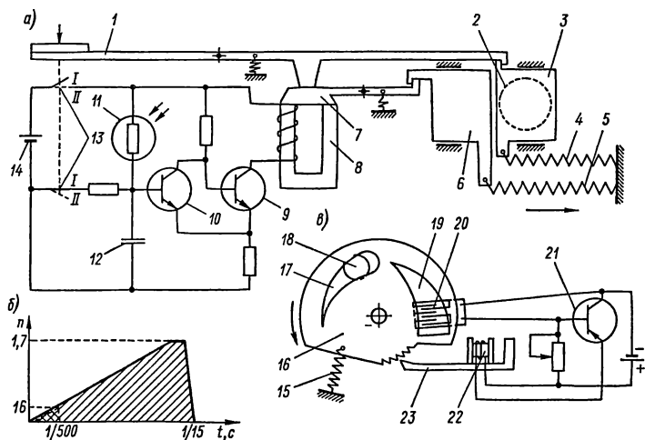
Рис. 40. Электронные фотозатворы: а — система автоматической установки выдержки; б — диаграмма работы программного затвора-диафрагмы; в — система автоматической установки диафрагмы
