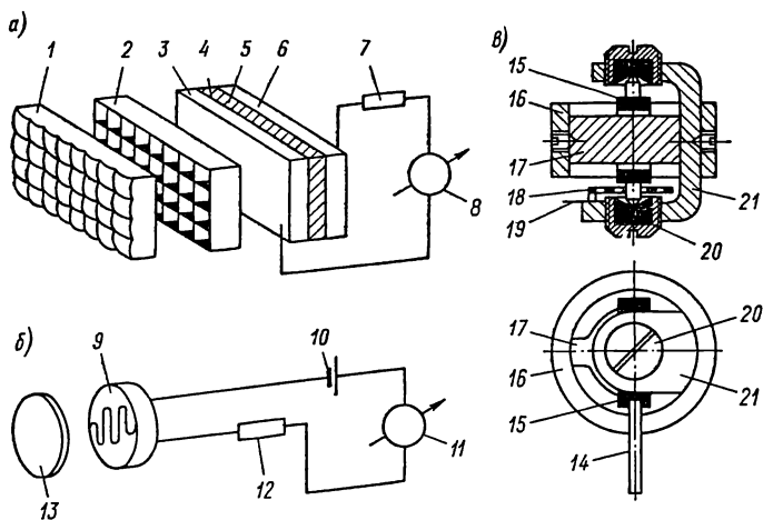
Рис. 32. Экспонетрические устройства: а — с селеновым фотоэлементом; б — с фоторезистором; в — гальванометр (разрез конструкции и вид сверху)
