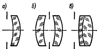
Рис. 4. Схемы простейших объективов: а — мениск; б — перископ; в — ахромат
