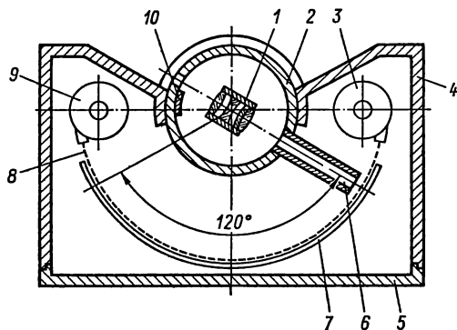
Рис. 15. Схема панорамного фотоаппарата. 1 — объектив; 2 — барабан с пружинным двигателем; 3 — подающая кассета; 4 — корпус; 5 — задняя крышка; 6 — щель; 7 — дугообразная прижимная планка; 8 — фотопленка; 9 — приемная кассета; 10 — заслонка, защищающая пленку от засветки
