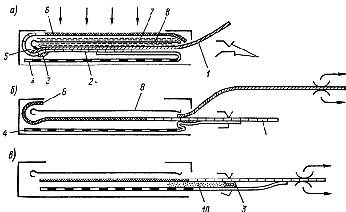
Рис. 50. Схема одноступенного фотопроявления в фильмпак:
