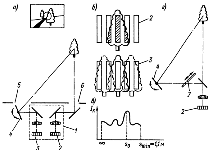
Рис. 45. Автофокусирующая система «Визитроник»: а — дальномерное поле в видоискателе и схема проецирования двух изображений на модуль; б — изображения на фотоприемниках при фокусировке; в — изменение корреляционного сигнала при автофокусировке; г — система с одним составным фотоприемником
