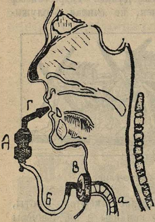
Схема действия искусственной гортани.
