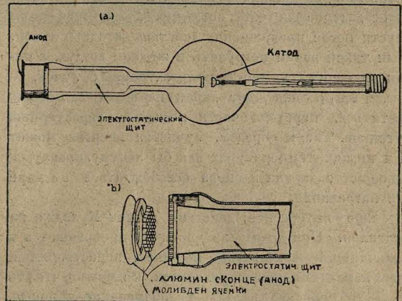
Схематический чертеж электронной пушки Кулиджа.
