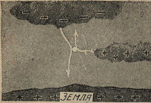
Рис. 6. Образование шаровой молнии в месте сближения двух молний обычного вида
