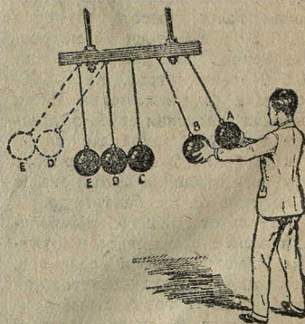
Опыты с упругими шарами
