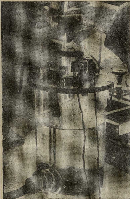
В лаборатории опытного поля. Прибор для определения электропроводности в почвенном растворе
