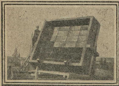
Установка солнечных опреснителей
