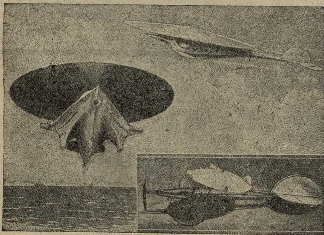
Аппарат с дискообразным вращающимся крылом, наполненным газом или нагретым воздухом. Внизу — снимок маленькой летающей модели такого аппарата.
