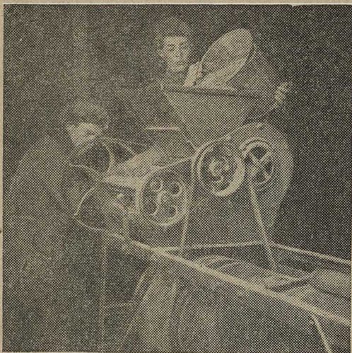
На снимке: работники совхоза „Большевик“ Серпуховского района за очисткой семян на триере для весеннего сева
