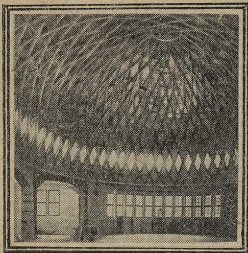
Замена металлического перекрытия деревянным в куполообразном здании Кобленца
