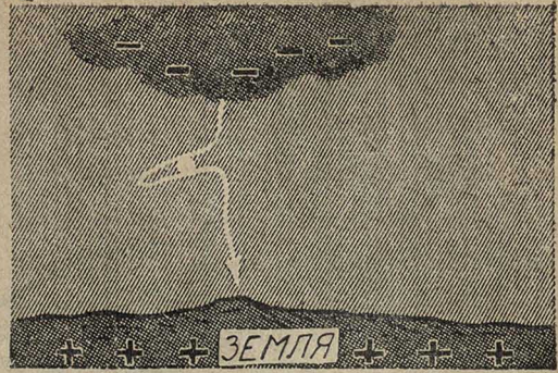
Рис. 7. Другой случай образования шаровой молнии
