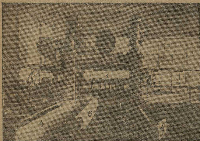
Рис. 3. Блюминг с валками европейского типа
