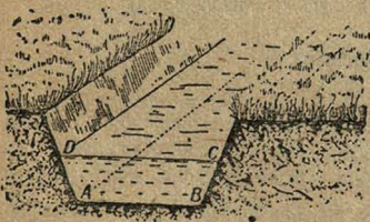
Вычисление расхода воды в канаве
