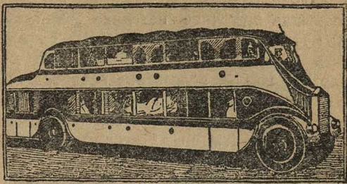
Рис. 4. Автобус Сан-Франциско — Лос-Анжелос. 28 мест, из них 8 спальных
