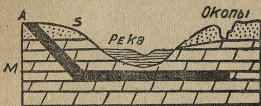
Подземная галерея под окопы противника. M—мергель, S—песок А—устье шахты
