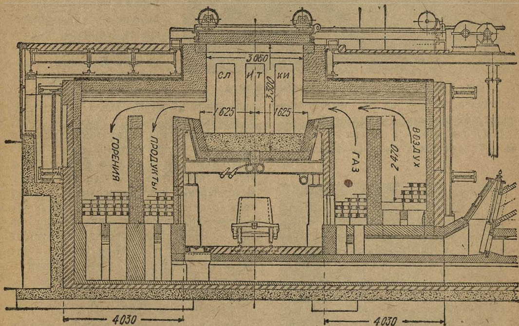
Рис. 2. Ячейка нагревательного колодца
