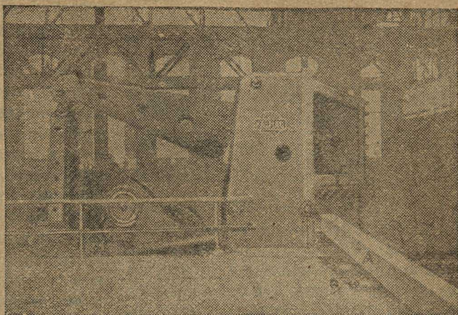
Рис. 5. Электрические ножницы для резки блюма
