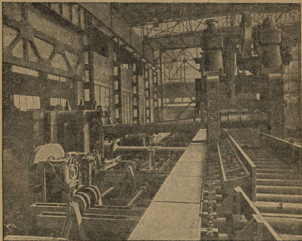
Блюминг с валками американского типа
