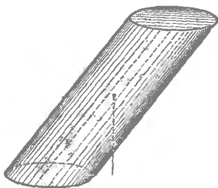
Рис. 14. Такой цилиндр должен опрокинуться, потому что отвесная линия, проведенная из центра тяжести, проходит вне основания.
