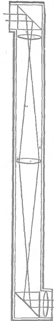
Рис. 97. Схема перископа подводной лодки.
