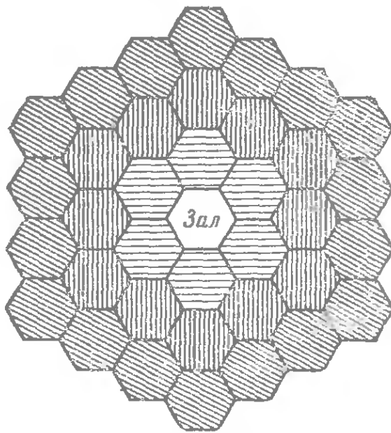
Рис. 106. Троекратное отражение стен центрального зала дает 36 зал.
