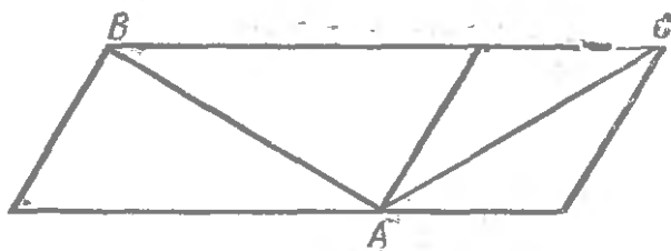
Рис. 144. Расстояния AB и AC равны, хотя первое кажется большим.
