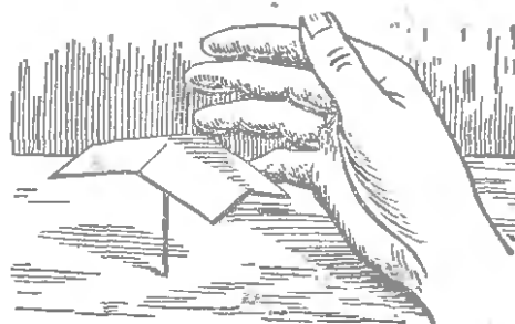
Рис. 82. Почему бумажка вертится?
