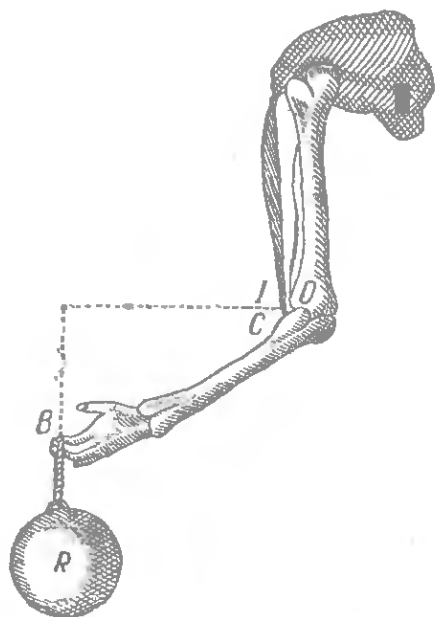
Рис. 27. Предплечье С человека — рычаг второго рода. Действующая сила приложена к точке I ; опора рычага находится в точке О сочленения; преодолеваемое же сопротивление (груз R ) приложено в точке В . Расстояние ВО больше расстояния IO приблизительно в 8 раз. (Рисунок взят из старинного сочинения Борелли, флорентийского ученого XVII века, «О движении животных», где законы механики впервые прилагаются к физиологии.)
