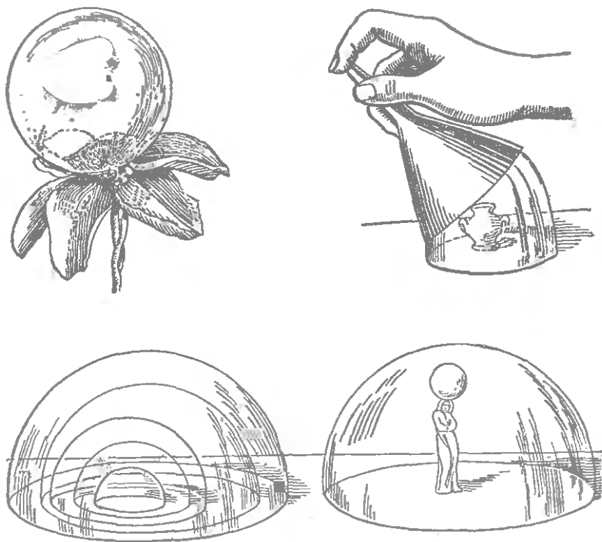
Рис. 66. Опыты с мыльными пузырями: пузырь на цветке; пузырь вокруг вазы; ряд пузырей друг в друге; пузырь на статуэтке внутри другого пузыря.
