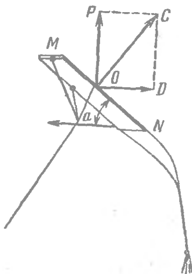
Рис. 31. Какие силы действуют на бумажный змей.
