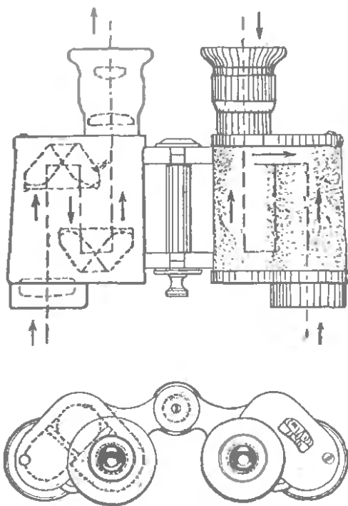
Рис. 132. Призмный бинокль.
