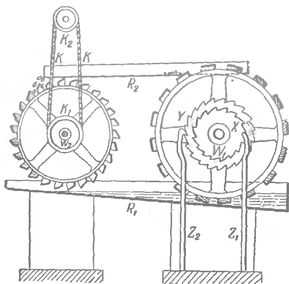
Рис. 77. Часы, которые заводятся сами собой.
