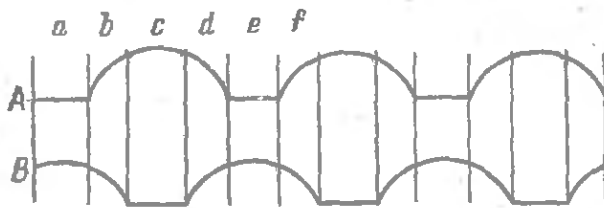
Рис. 20. Графическое изображение движения ног в беге (ср. с рис. 18). Из графика видно, что для бегущего человека существуют моменты (b, d, f), когда обе ноги витают в воздухе. Этим и отличается бег от ходьбы.
