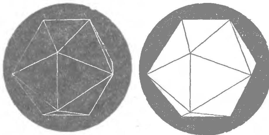
Рис. 133. Стереоскопический блеск. Сливаясь при рассмотрении в стереоскоп, эти рисунки дают изображение блестящего кристалла на черном фоне.
