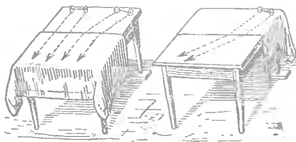
Рис. 109. Опыт, поясняющий преломление света.
