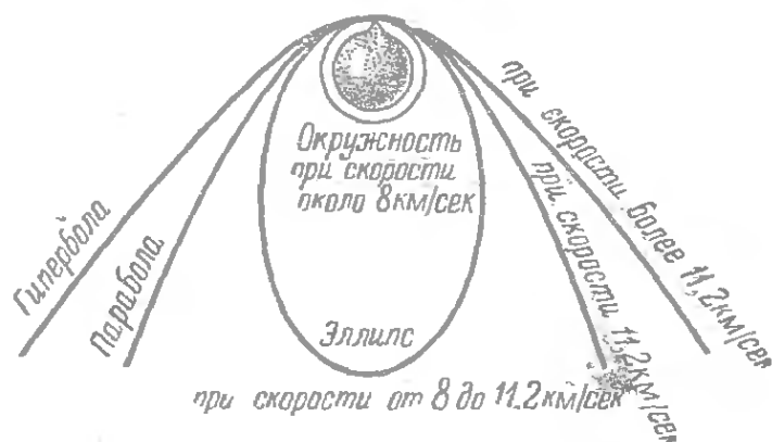
Рис. 26. Судьба пушечного снаряда, выпущенного с начальной скоростью 8 \text{ км/сек} и более.
