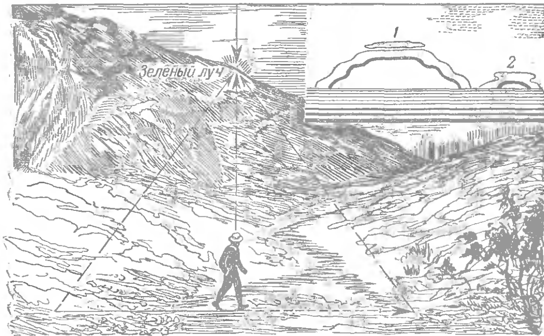
Рис. 119. Длительное наблюдение «зеленого луча»; наблюдатель видел «зеленый луч» за горным хребтом в течение 5 минут. Выше справа — «зеленый луч», видимый в подзорную трубу. Диск Солнца имеет неправильные контуры. В положении 1 блеск солнечного диска ослепляет глаз и мешает видеть зеленую каемку простым глазом. В положении 2, когда диск Солнца почти исчезает, «зеленый луч» становится доступным простому глазу.
