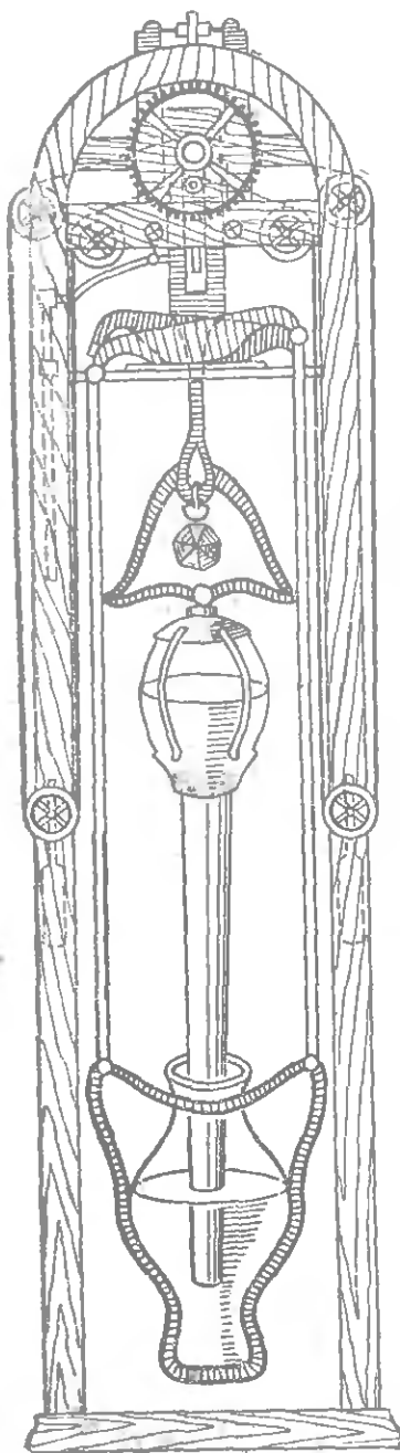
Рис. 72. Устройство дарового двигателя XVIII в.
