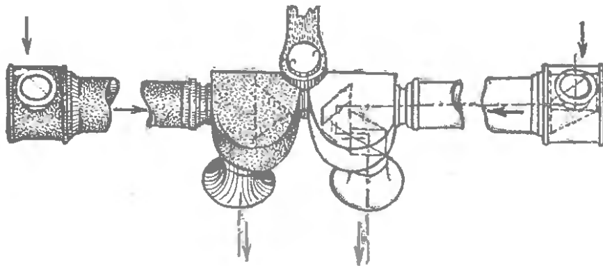
Рис. 131. Стереоскопическая зрительная труба.
